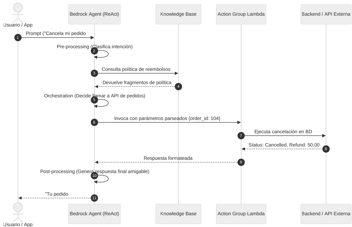
Ciclo de vida de una invocación a un Amazon Bedrock Agent: pre-processing, orquestación (ReAct) con Knowledge Base y Action Group, y post-processing.
