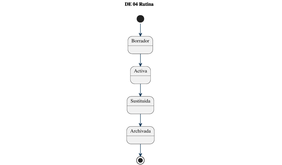
Figura 68: Estados de la rutina.
