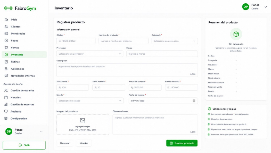
Figura 15: MU-28: Registro de producto y stock minimo. Rol: Dueño/Administrador. RF: RF-INV-01.
