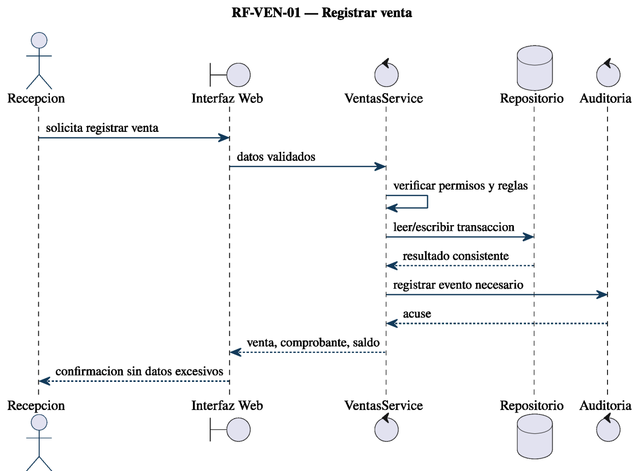
Figura 55: Diagrama de secuencia de RF-VEN-01: registrar venta.
