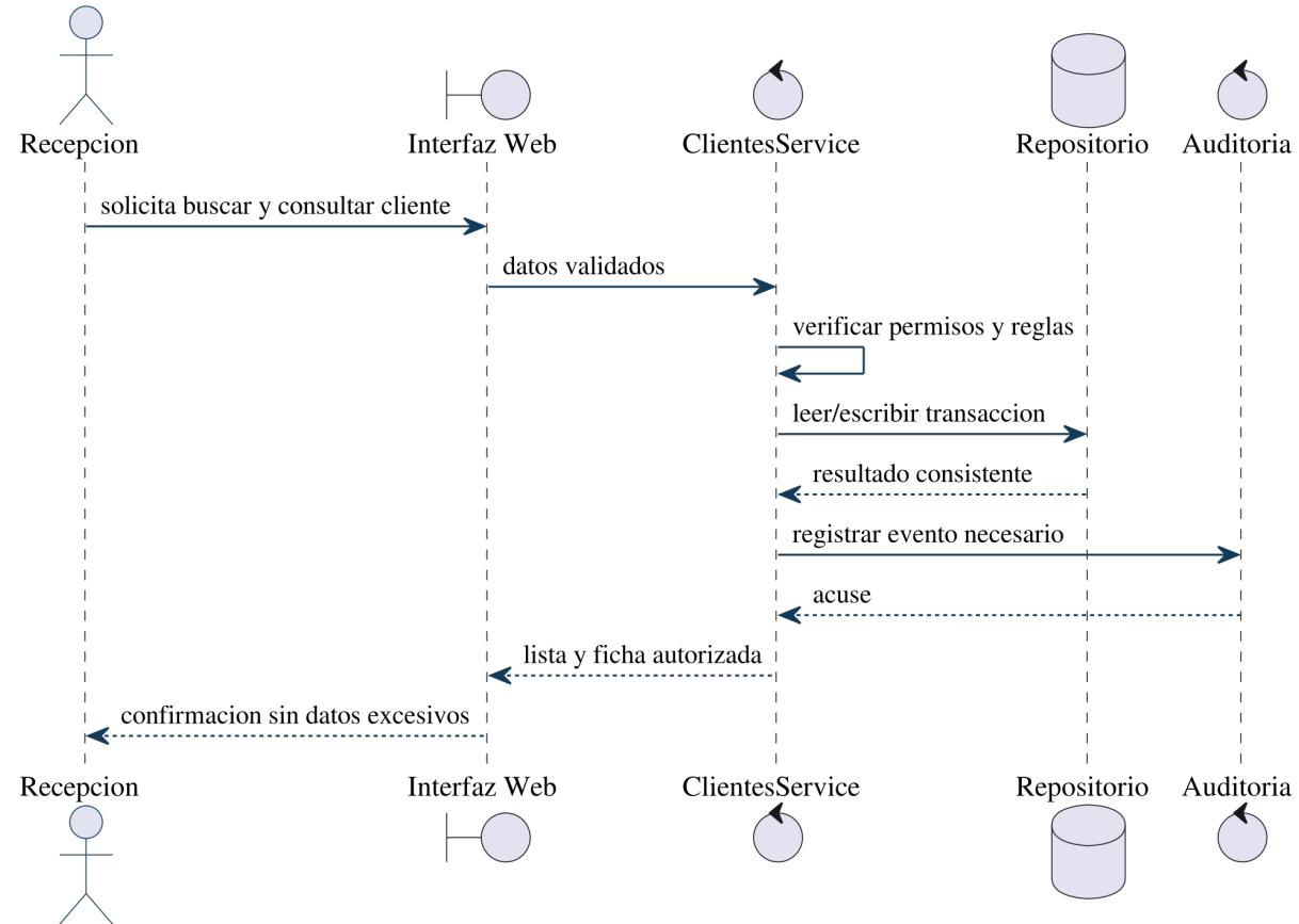
Figura 44: Diagrama de secuencia de RF-CLI-02: buscar y consultar cliente.
