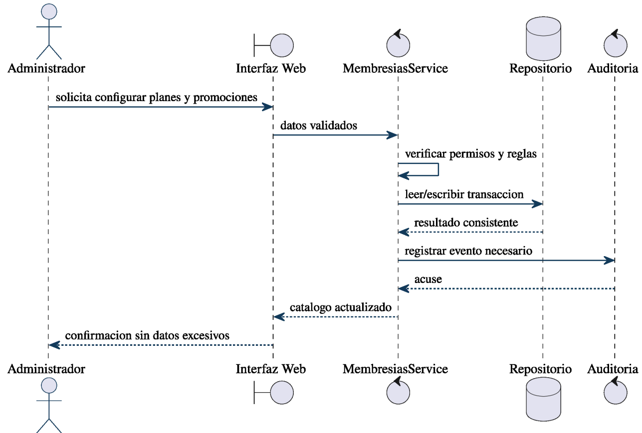
Figura 46: Diagrama de secuencia de RF-MEM-01: configurar planes y promociones.
