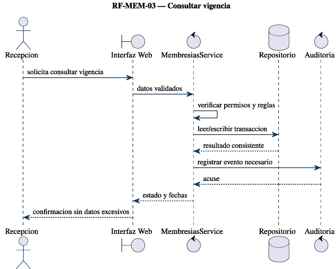
Figura 48: Diagrama de secuencia de RF-MEM-03: consultar vigencia.
