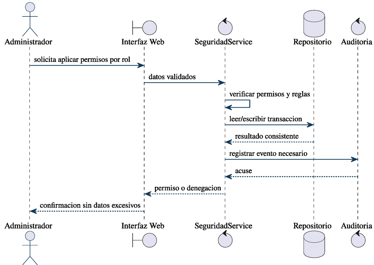
Figura 42: Diagrama de secuencia de RF-AUT-02: aplicar permisos por rol.
