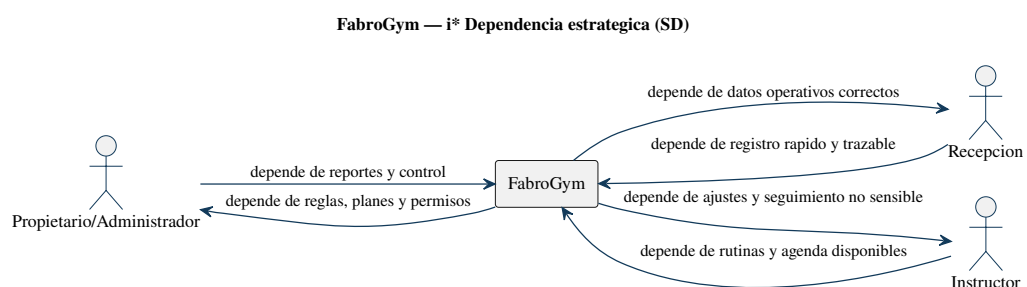
Figura 3: Dependencias estratégicas (SD).
