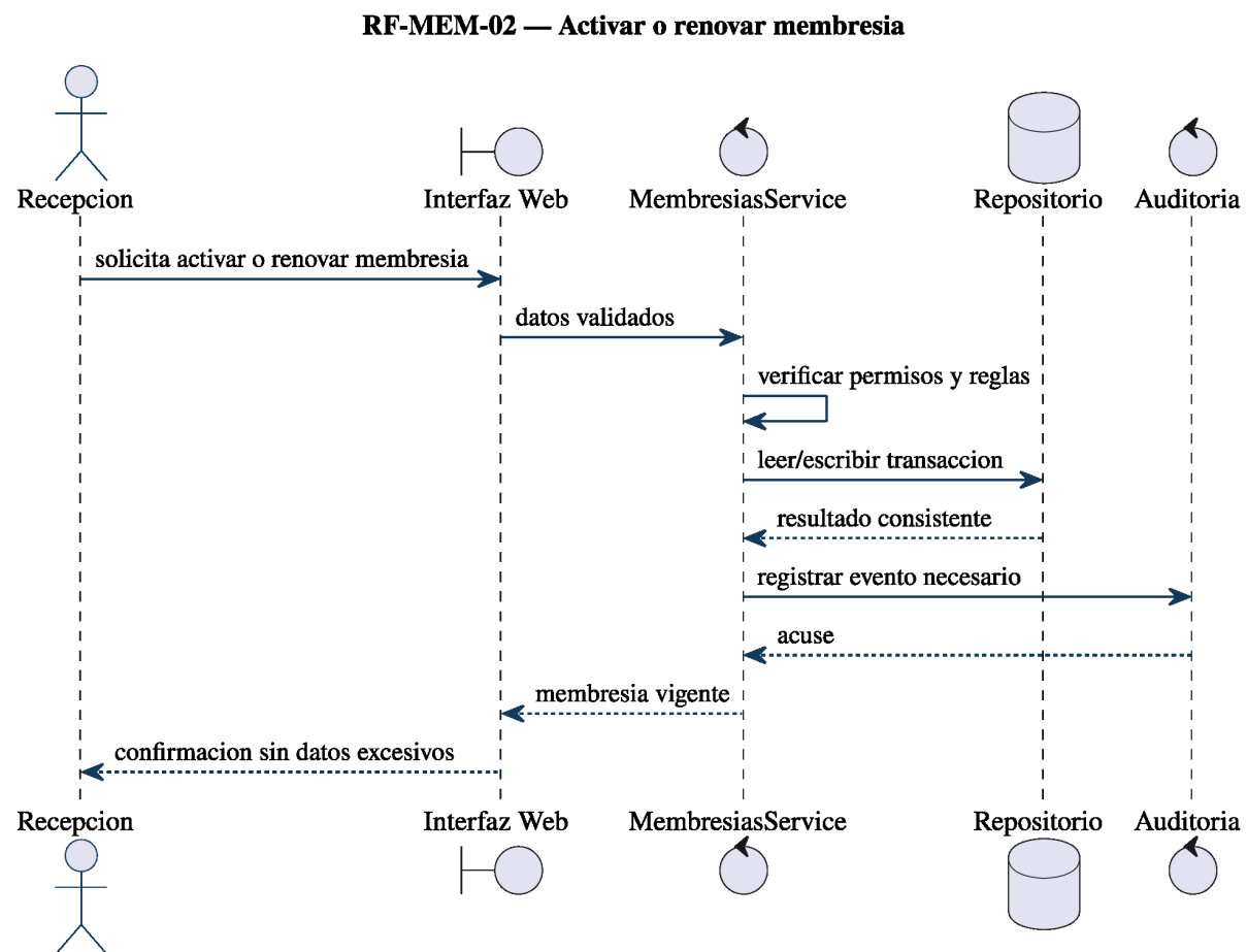
Figura 47: Diagrama de secuencia de RF-MEM-02: activar o renovar membresia.
