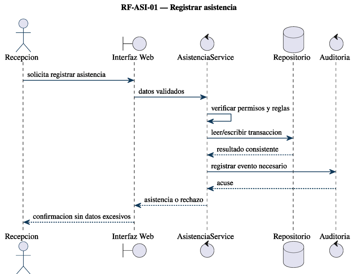
Figura 51: Diagrama de secuencia de RF-ASI-01: registrar asistencia.
