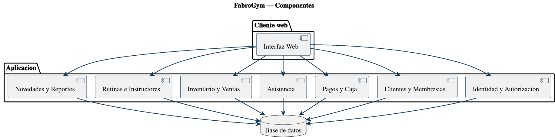
Figura 69: Componentes propuestos.
