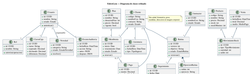
Figura 40: Clases refinadas.
