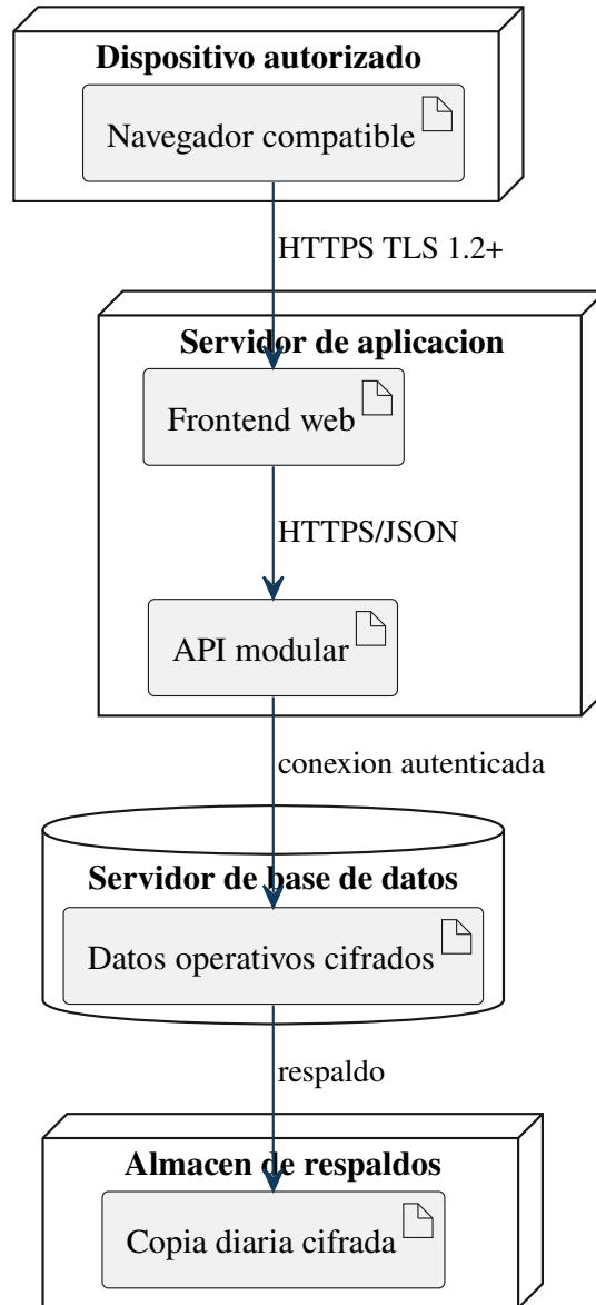
Figura 70: Despliegue propuesto.
