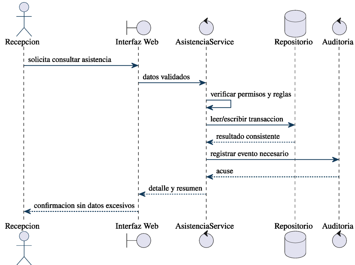
Figura 52: Diagrama de secuencia de RF-ASI-02: consultar asistencia.
