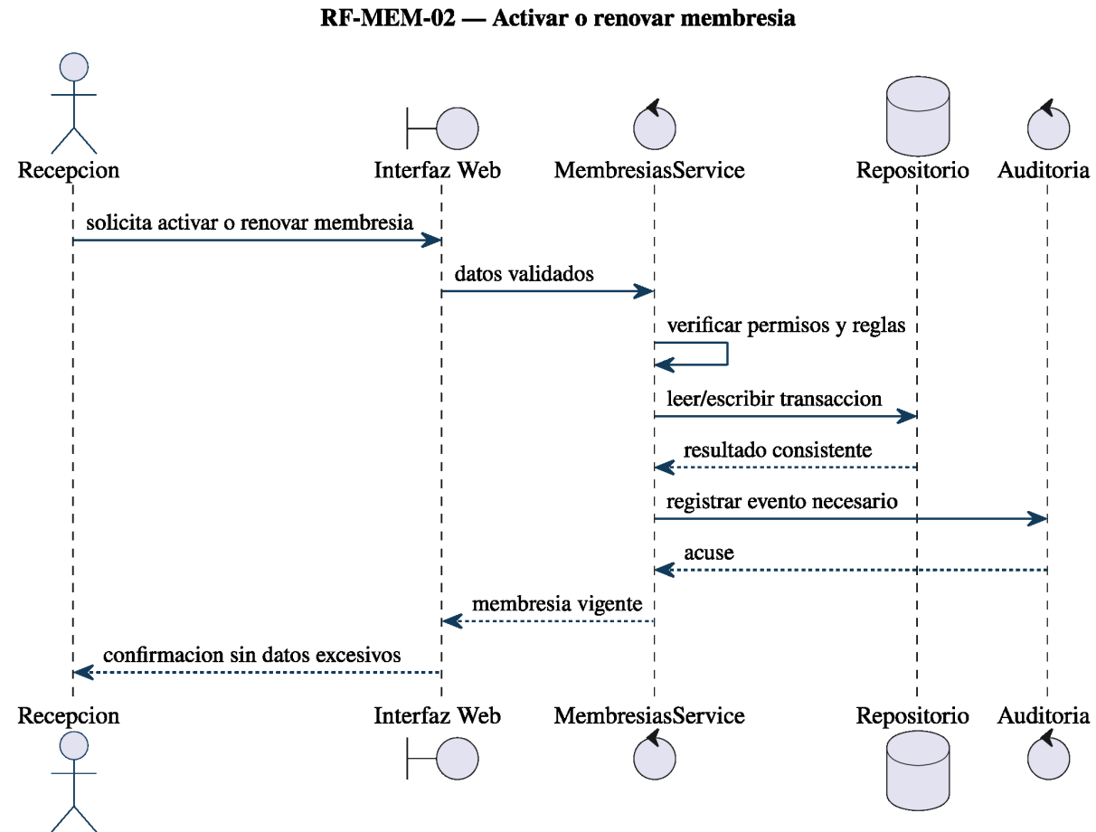
Figura 47: Diagrama de secuencia de RF-MEM-02: activar o renovar membresia.
