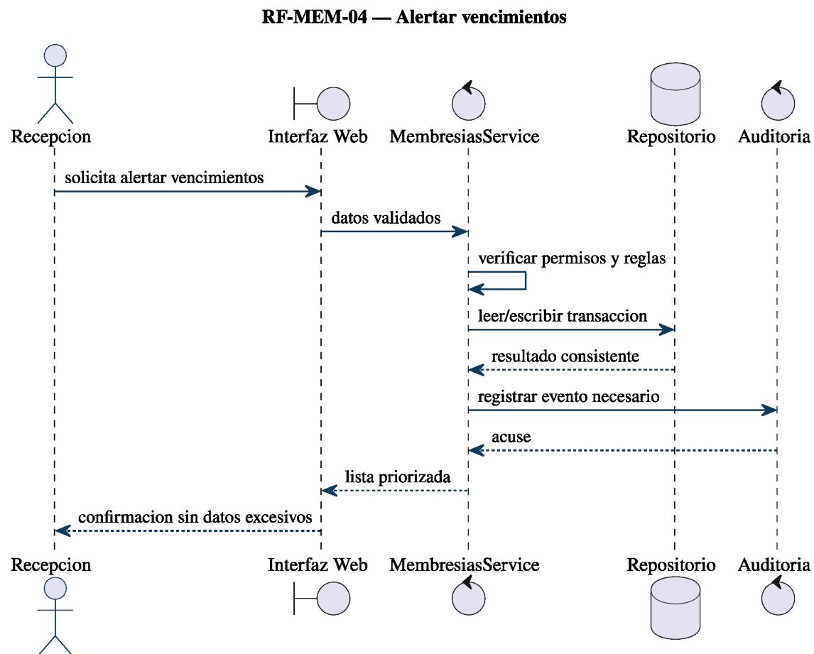
Figura 49: Diagrama de secuencia de RF-MEM-04: alertar vencimientos.
