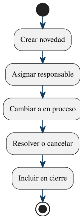
Figura 64: Actividad de novedad y turno.
