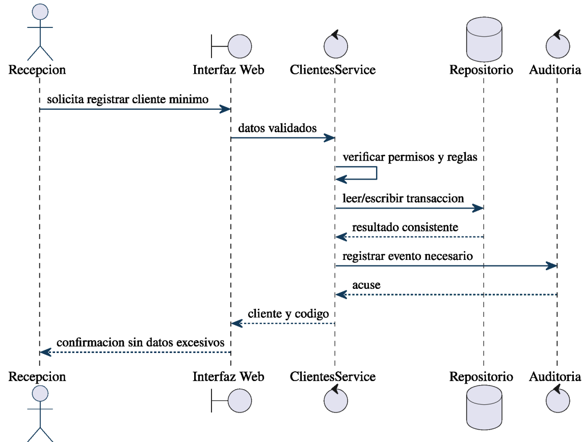
Figura 43: Diagrama de secuencia de RF-CLI-01: registrar cliente minimo.
