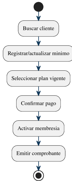
Figura 60: Actividad de alta o renovacion de membresia.
