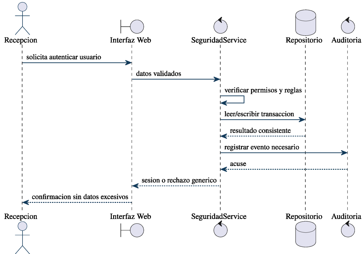
Figura 41: Diagrama de secuencia de RF-AUT-01: autenticar usuario.
