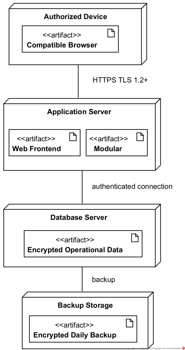
Figura 8: Diagrama de despliegue definitivo.
