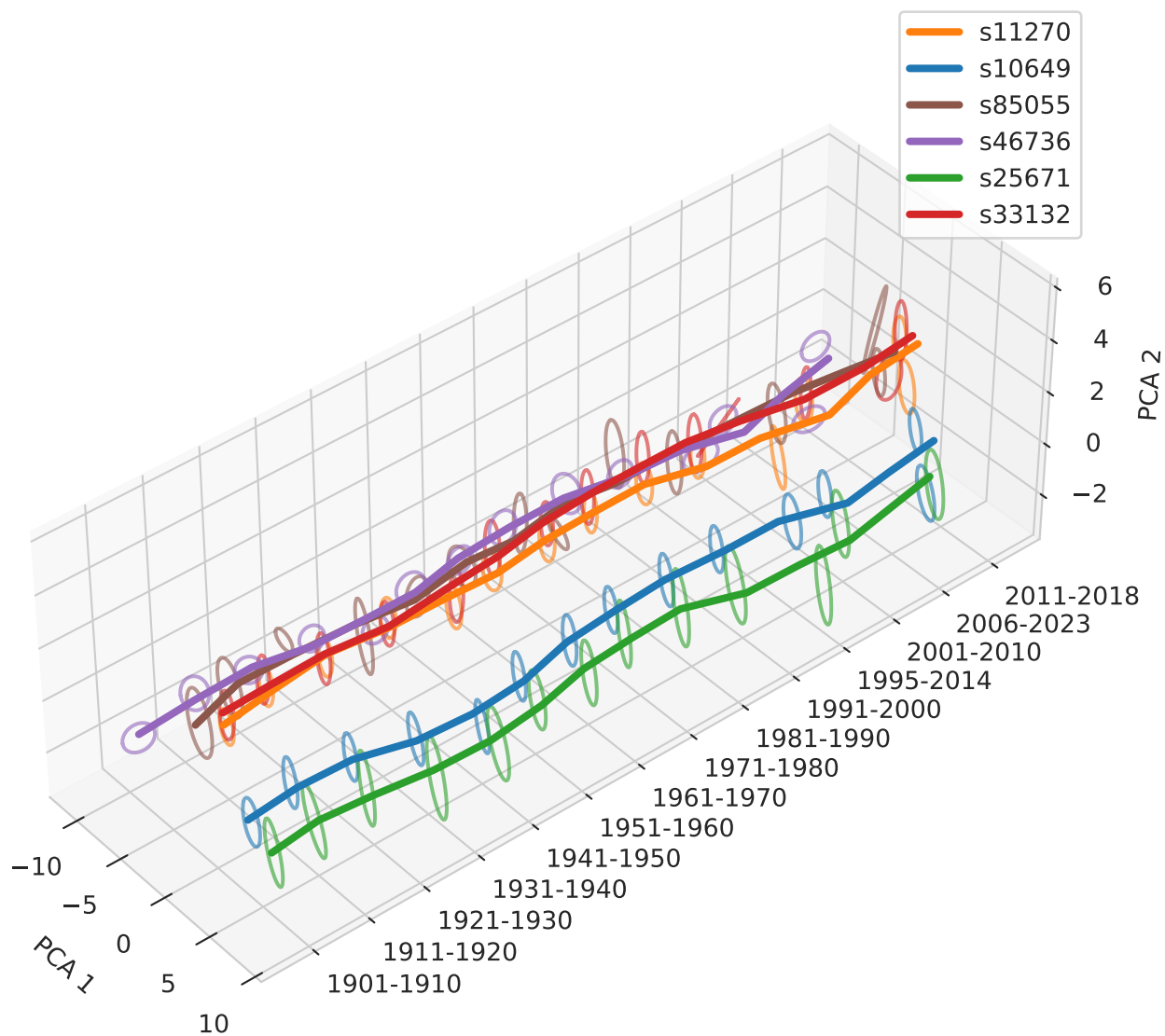
blatt: Sense Trajectories (PCA)
