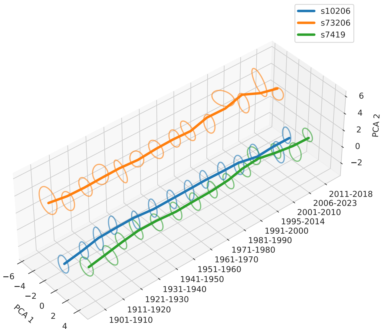
decke: Sense Trajectories (PCA)
