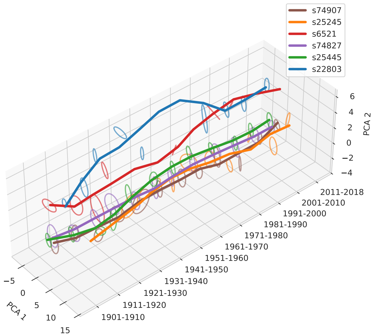
kasse: Sense Trajectories (PCA)
