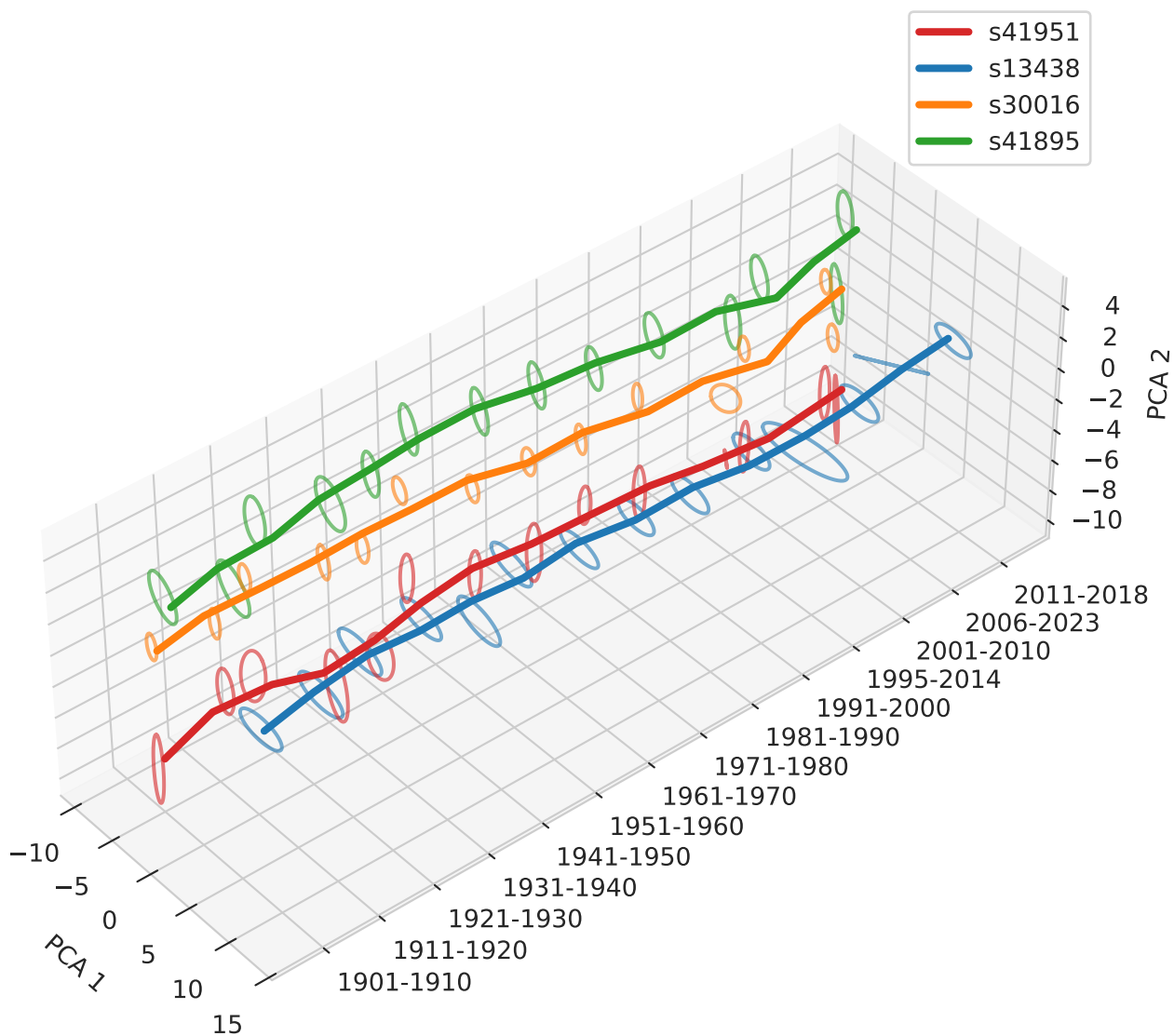
kurs: Sense Trajectories (PCA)
