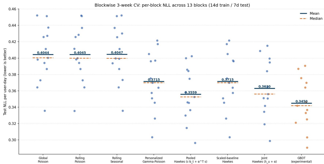
Figure 12: Поблочная CV: per-block NLL
