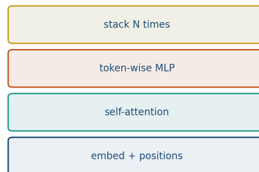
Encoder (BERT)
