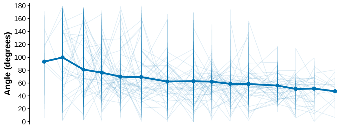
NN2
