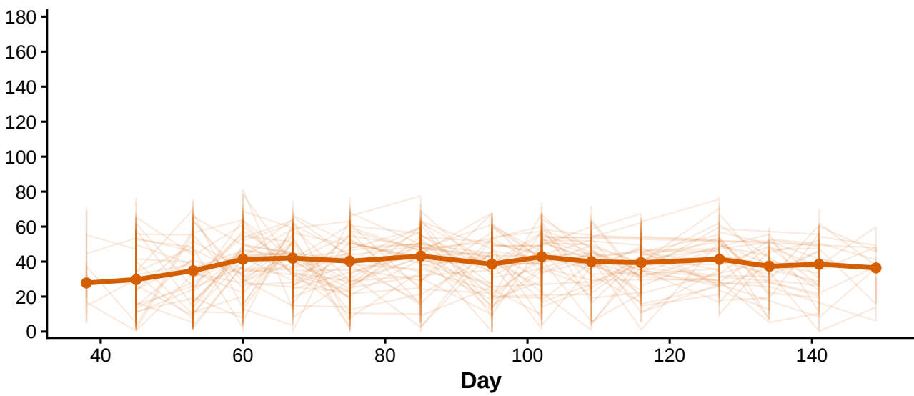
NN2
