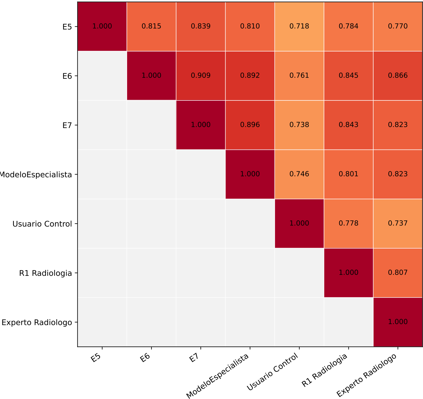
Matriz IoU > \epsilon
