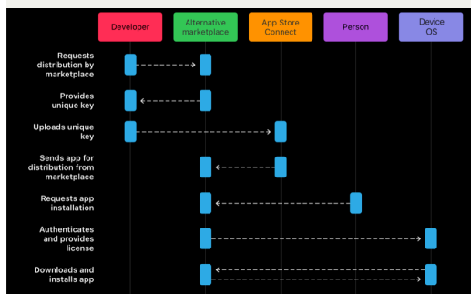
Apple Cork Lab 이후 정리한 설치 Flow와 iOS 아키텍처 초안
