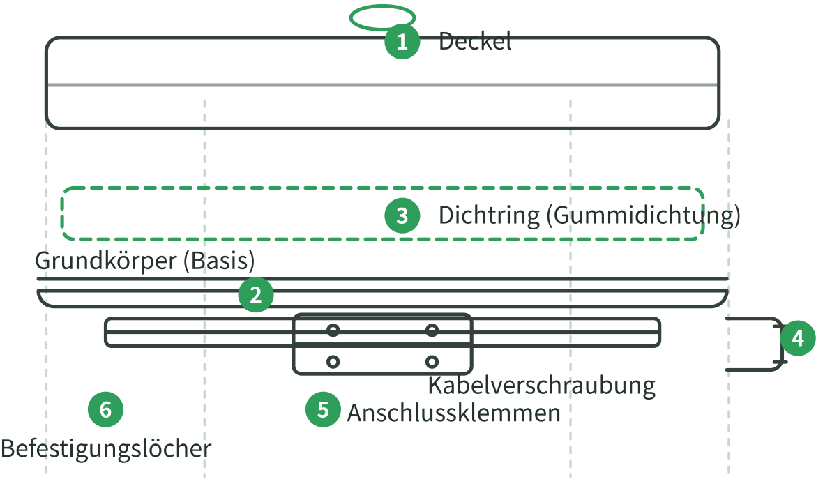
Abb. 2 — Bauteile: ① Deckel • ② Grundkörper • ③ Dichtring • ④ Kabelverschraubung • ⑤ Klemmen • ⑥ Befestigungslöcher
