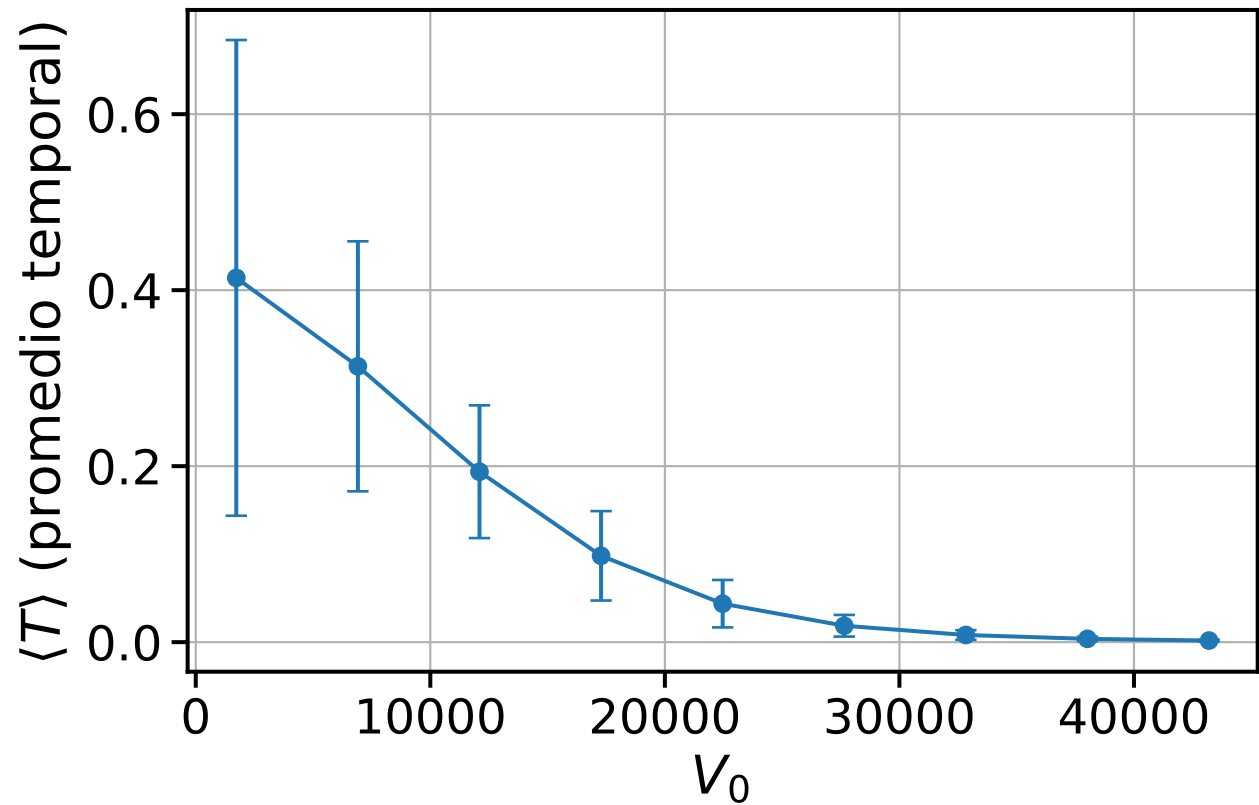
Transmisión media vs altura de barrera
