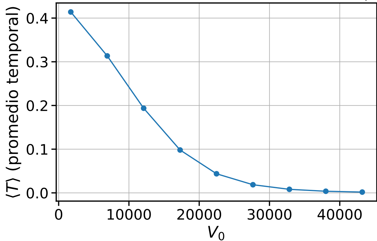
Transmisión media vs altura de barrera (sin \sigma )
