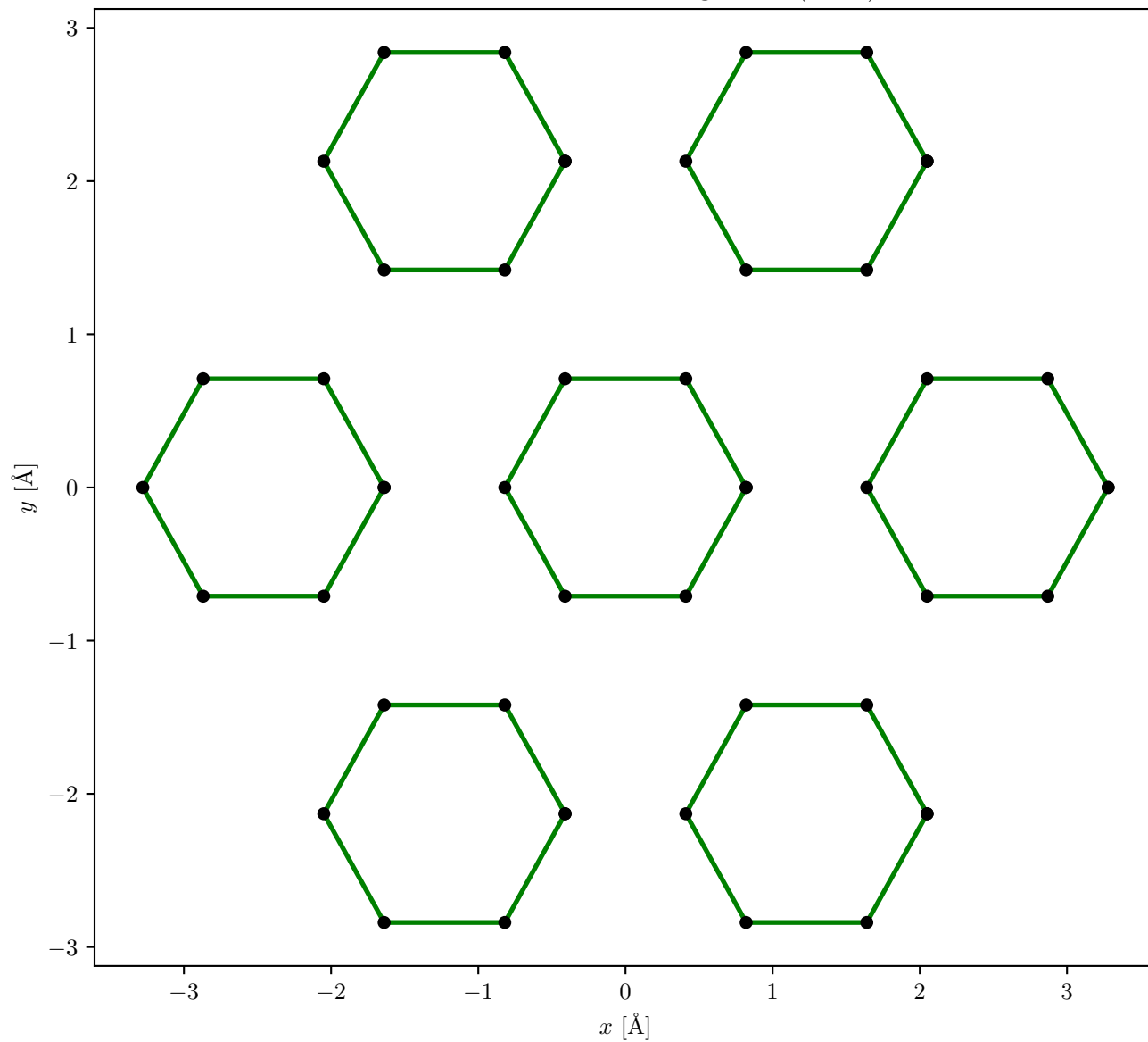
Estructura Atómica: Nanografeno (HBC)
