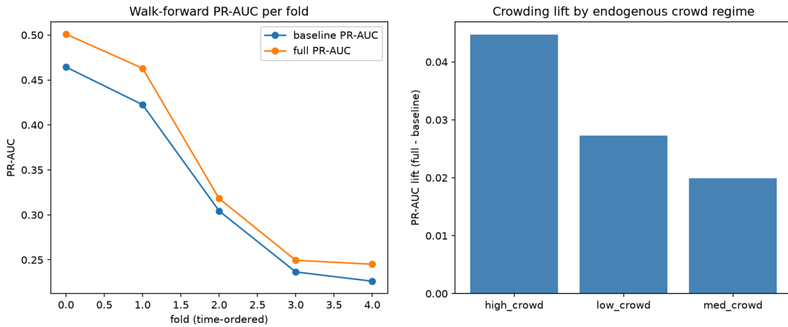
Hình 12: Walk-forward xoay vòng và độ bền theo chế độ thị trường (Phần 11). Trái: PR-AUC theo fold cho mô hình nền và mô hình đầy đủ LightGBM qua năm fold của sổ mở rộng của Bảng 5. Phải: mức tăng PR-AUC (đầy đủ – nền) theo chế độ đông đúc nội sinh, từ Bảng 6.
