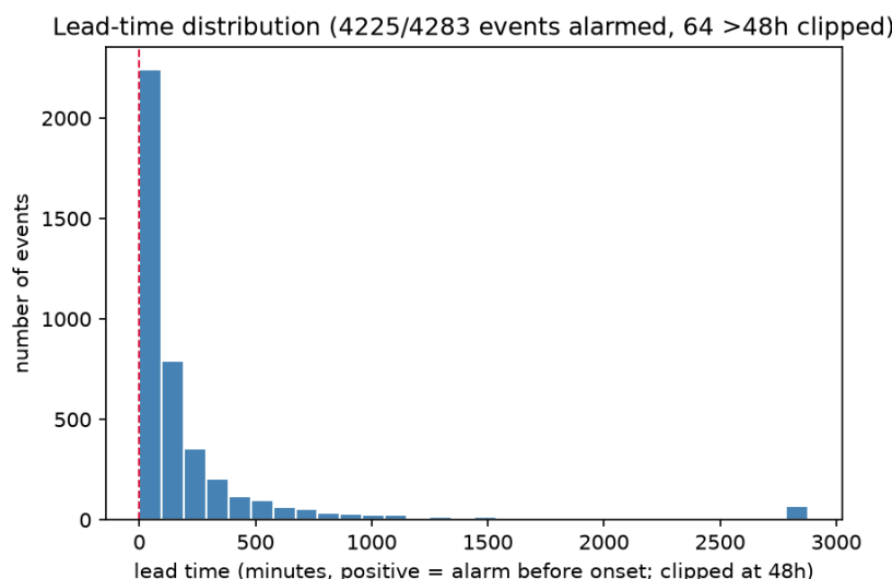
Hình 10: Phân phối thời gian cảnh báo sớm qua 4.225 sự kiện sụp đổ được cảnh báo (cắt tại 48h; 64 sự kiện vượt ngưỡng này là trạng thái cảnh báo liên tục, không phải cảnh báo rời rạc). Trung vị 90 phút, p10 10 phút, p90 570 phút.
