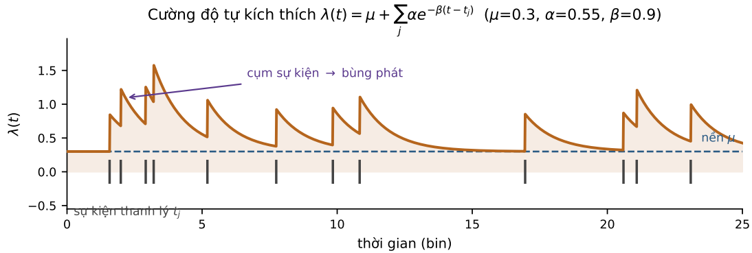
Hình 1: Ví dụ minh họa đường cường độ Hawkes tự kích thích (mô phỏng; \mu = 0,3, \alpha = 0,55, \beta = 0,9 , tỷ lệ phân nhánh \frac{\alpha}{\beta} \approx 0,61 ). Các vạch đứng là thời điểm sự kiện mô phỏng; đường cong là \lambda(t) . Mỗi sự kiện kích hoạt một bước nhảy tức thời độ lớn \alpha rồi suy giảm mũ với tốc độ \beta ; một cụm sự kiện gần nhau cộng dồn các bước nhảy này thành một đợt bùng phát rõ rệt trước khi \lambda(t) hạ về lại mức nền \mu (nét đứt).
