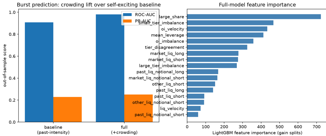
Hình 11: Dự báo bùng phát trên giai đoạn kiểm tra theo thời gian, an toàn không rò rỉ. Trái: ROC-AUC và PR-AUC ngoài mẫu cho mô hình nền LightGBM tự kích thích so với mô hình đầy đủ đã tinh chỉnh. Phải: mức độ quan trọng của đặc trưng LightGBM của mô hình đầy đủ. Xem Bảng 4 để so sánh đầy đủ.
