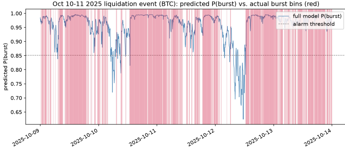
Hình 7: P (bùng phát) dự đoán cho BTC xuyên suốt sự kiện ngày 10–11/10/2025 (890 khung bùng phát trong cửa sổ), mô hình chỉ được huấn luyện trên dữ liệu trước ngày 7/10/2025. Đường đỏ đánh dấu khung bùng phát thực tế; đường đứt nét là ngưỡng cảnh báo (điểm số top-5% của tập huấn luyện). Cảnh báo đầu tiên của mô hình trên BTC đến trước khung bùng phát thực tế đầu tiên 20 phút.
