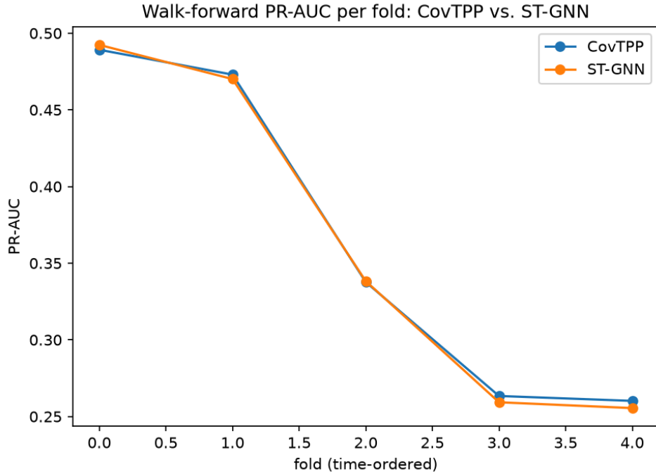
Hình 8: PR-AUC theo fold, CovTPP so với ST-GNN, qua cùng năm fold walk-forward như Hình 12. Hai đường gần như trùng khít nhau ở mọi fold.
