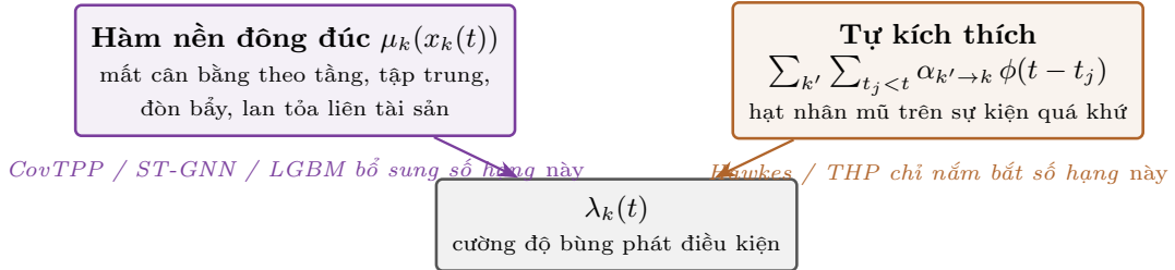
Hình 2: Phân rã cường độ bùng phát, Phương trình 4. Các mô hình nền đã công bố chỉ mô hình hóa số hạng tự kích thích (phải); các mô hình sử dụng hiệp biến trong luận văn này cung cấp hàm nền điều kiện hóa theo đồng đúc (trái). Luận văn đo mức tăng khi bổ sung số hạng bên trái, được tách bạch rõ nhất trong họ TPP thần kinh (THP \rightarrow CovTPP).
