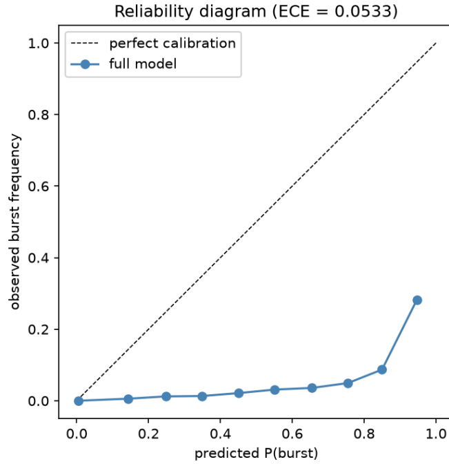
Hình 9: Biểu đồ độ tin cậy, mô hình LightGBM đầy đủ, dự đoán ngoài mẫu walk-forward gộp, 10 khoảng đều nhau. ECE = 0,0533; đường cong dưới đường chéo cho thấy sự quá tự tin có hệ thống.
