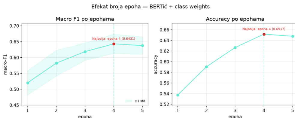
Слика 3.19 — Ефекат броја епоха на macro-F1 и accuracy — BERTuћ + class weights
