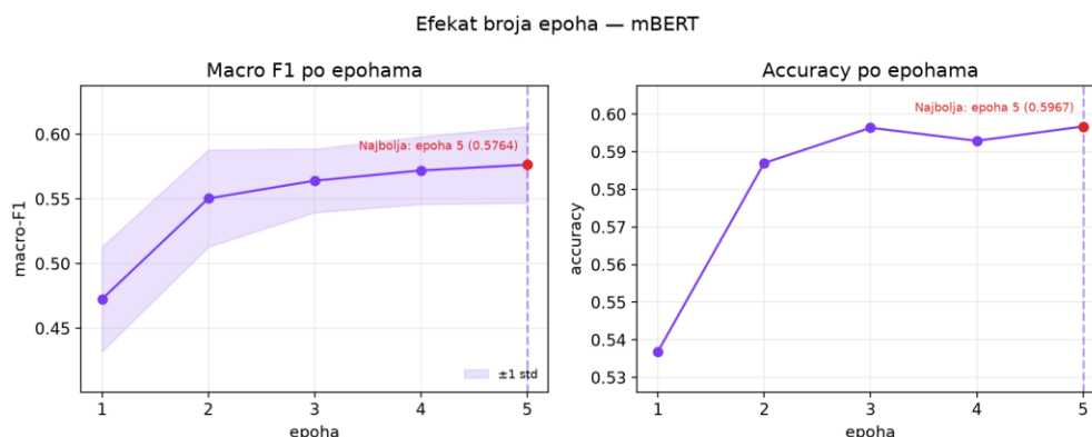
Слика 3.20 — Ефекат броја епоха на macro-F1 и accuracy — mBERT
