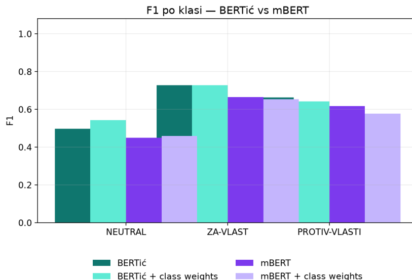
Слика 3.10 — F1 по класама, BERTić наспрам mBERT (све четири конфигурације)
