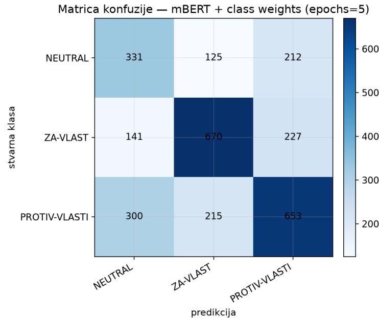
Слика 3.15 — Матрица конфузије за mBERT + class weights (epochs = 5)
