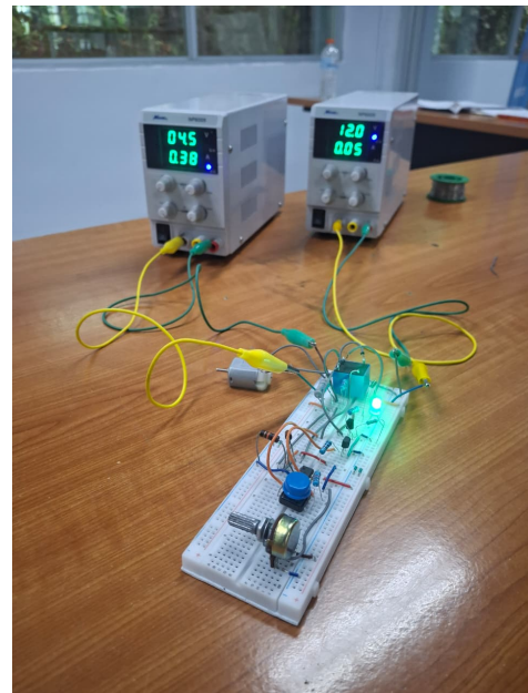
Fig. 5. Montaje físico del circuito en protoboard
