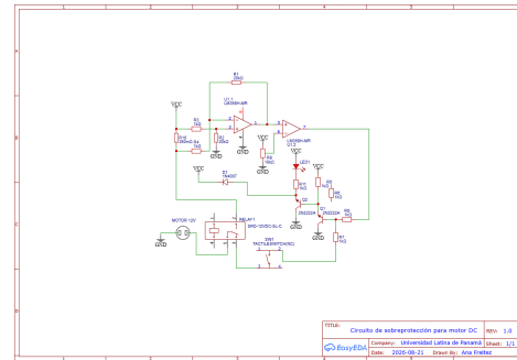
Fig. 4. Esquemático diseñado en EasyEDA
