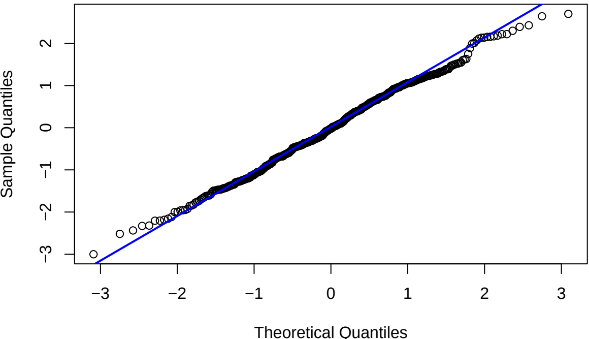
QQ Plot – Distribuição Normal
