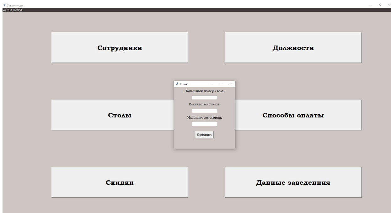
Рисунок 2.30 – Окно «Столы»
