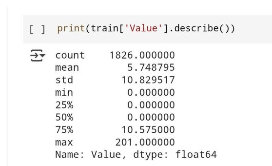
Figura 1 - Descrição estatística da coluna 'Value':
