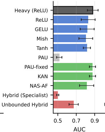
EEG Eye State
