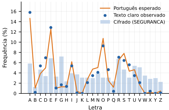
(a) Frequências antes e depois da cifra
