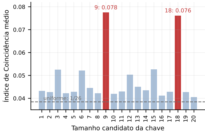
(b) IC médio por período candidato
