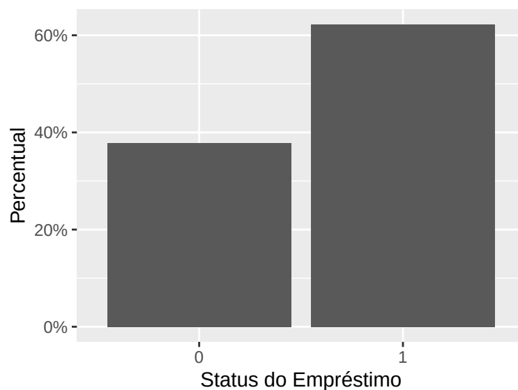
Figura 7: Distribuição da aprovação de empréstimos
