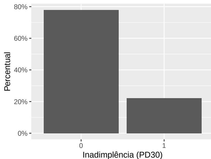
Figura 12: Distribuição da Inadimplência
