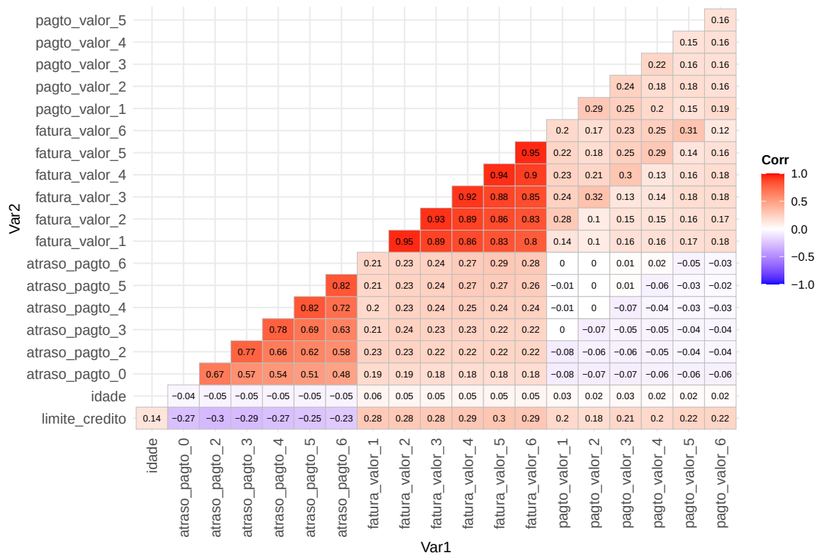
Figura 13: Mapa de calor da correlação entre variáveis numéricas do conjunto de dados de crédito
