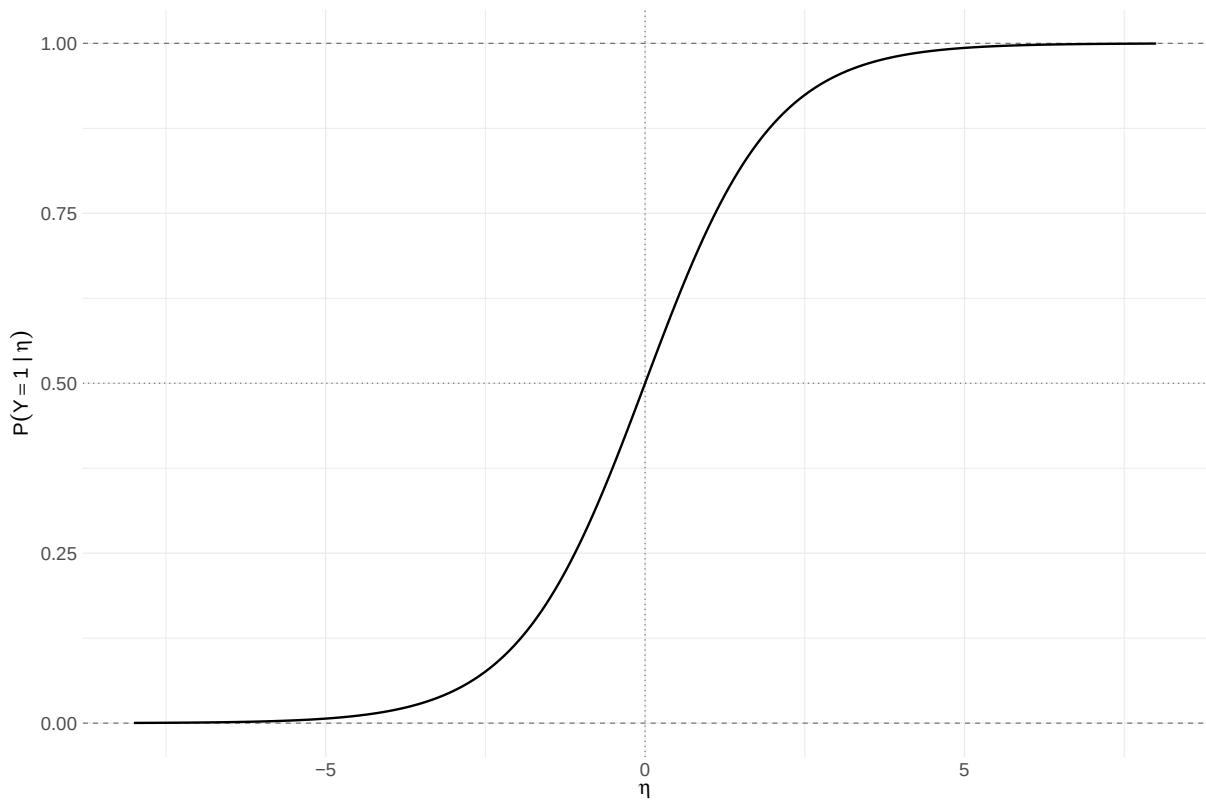
Figura 1: Função logística para um modelo com uma única variável preditora ( \beta_0 = 0 e \beta_1 = 1 ).
