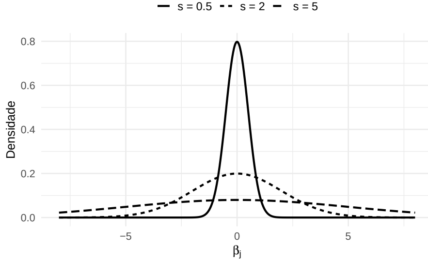
Figura 3: Distribuições Normais a priori com diferentes desvios padrão.
