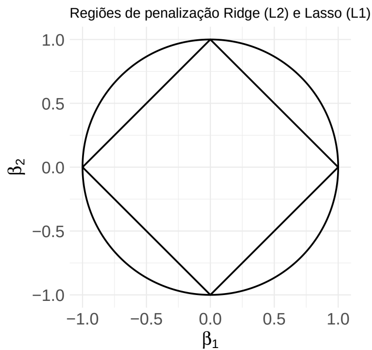
Figura 2: Representação geométrica das regiões de penalização Ridge (L2) e Lasso (L1). A região circular associada à penalização L2 tende a reduzir simultaneamente a magnitude dos coeficientes, enquanto a região em formato de losango da penalização L1 favorece soluções em que alguns coeficientes assumem valor exatamente igual a zero.
