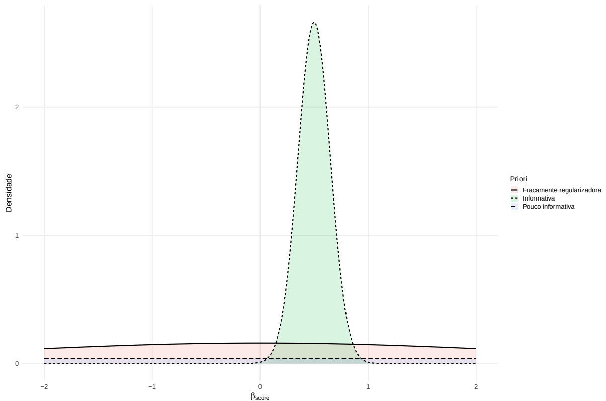
Figura 16: Diferentes distribuições a priori consideradas para o coeficiente associado ao score de crédito.
