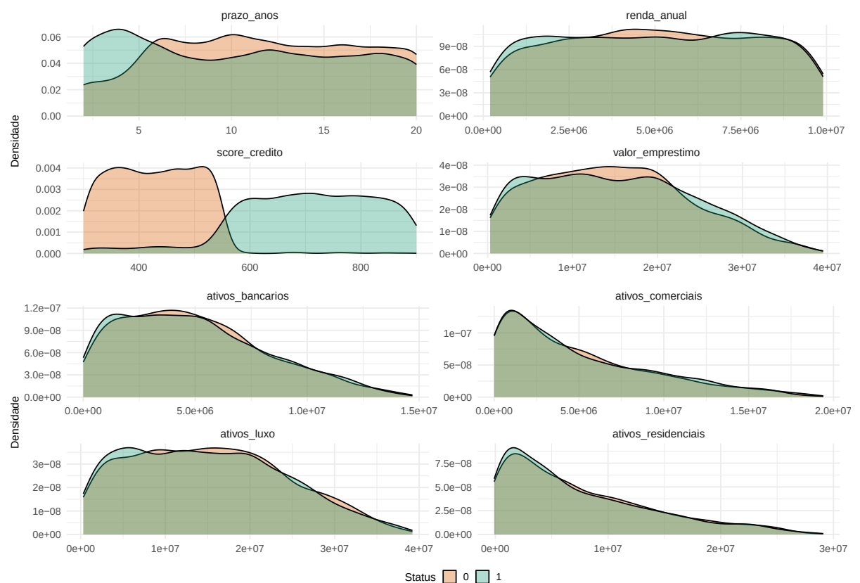
Figura 8: Distribuição das variáveis numéricas por status de aprovação do empréstimo
