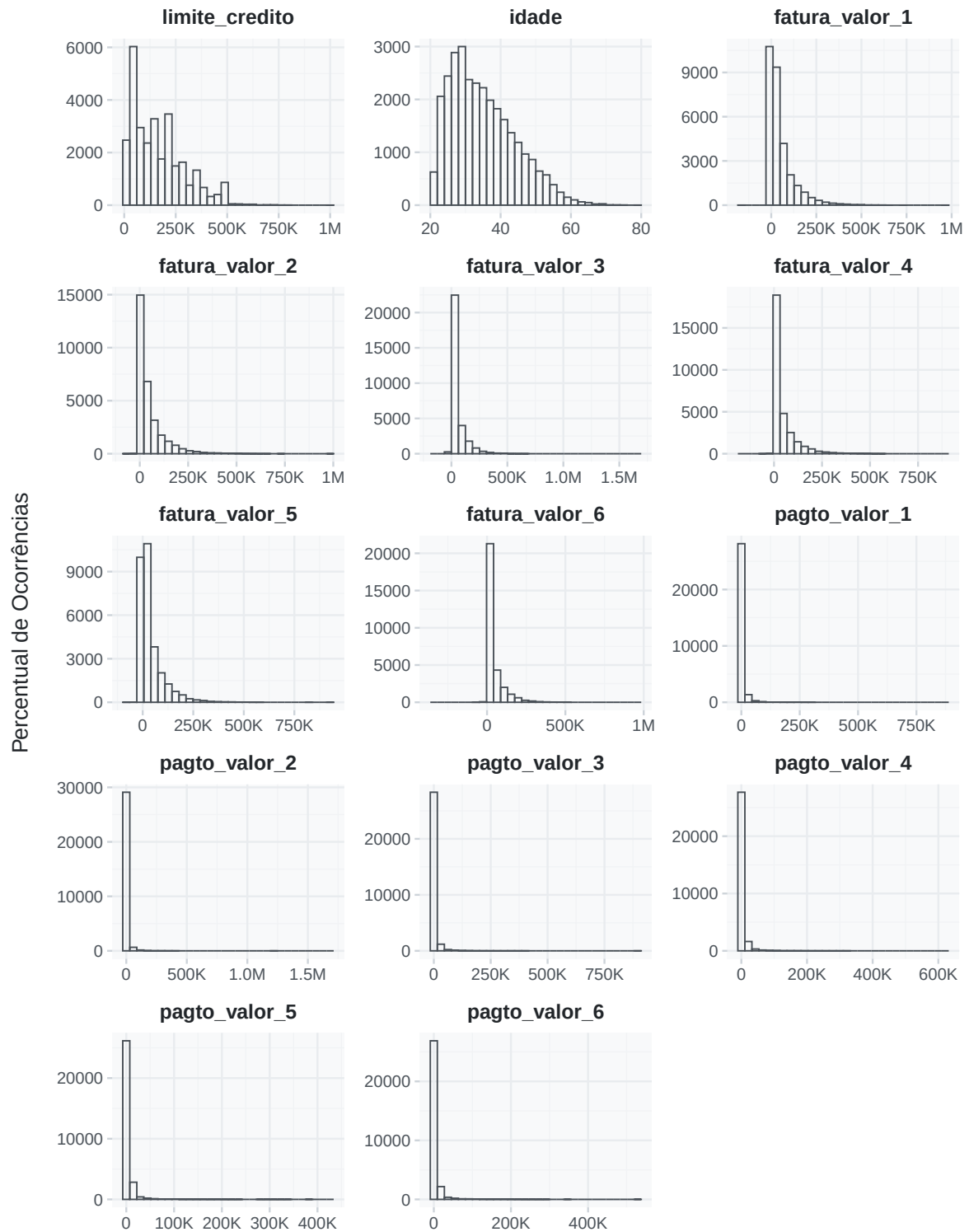
Figura 11: Distribuição das principais variáveis numéricas do conjunto de dados
