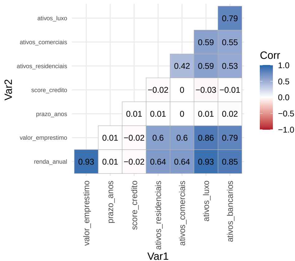
Figura 10: Mapa de calor da correlação entre variáveis numéricas
