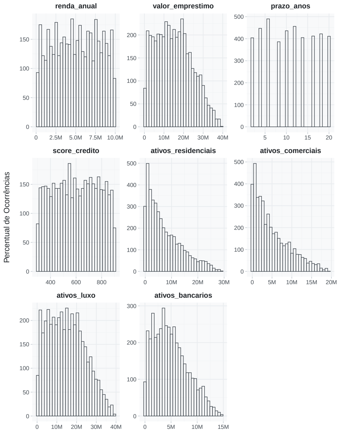
Figura 6: Distribuição das principais variáveis numéricas do conjunto de dados
