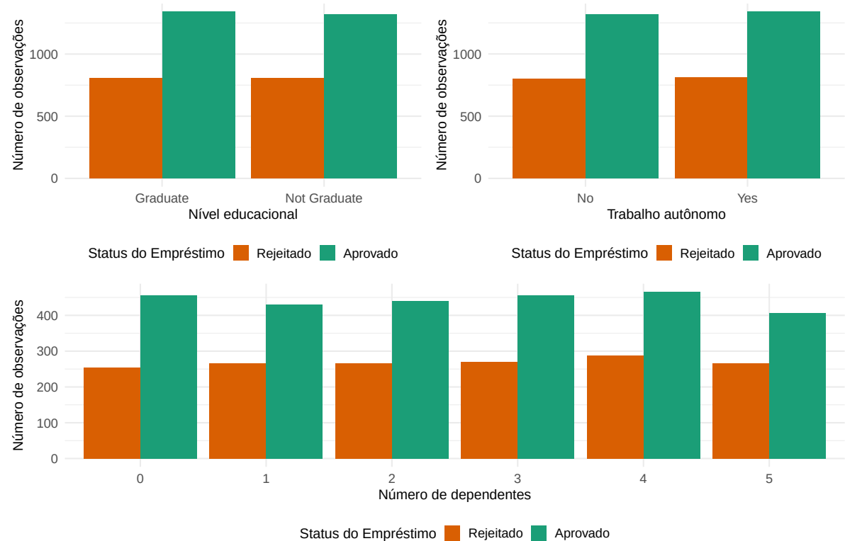
Figura 9: Distribuição das variáveis categóricas segundo o status do empréstimo
