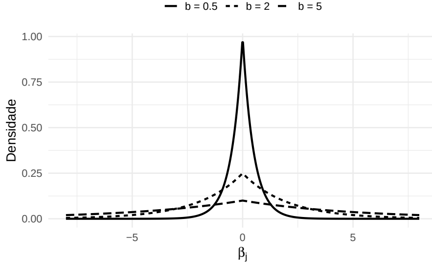
Figura 4: Distribuições Laplace a priori com diferentes parâmetros de escala.
