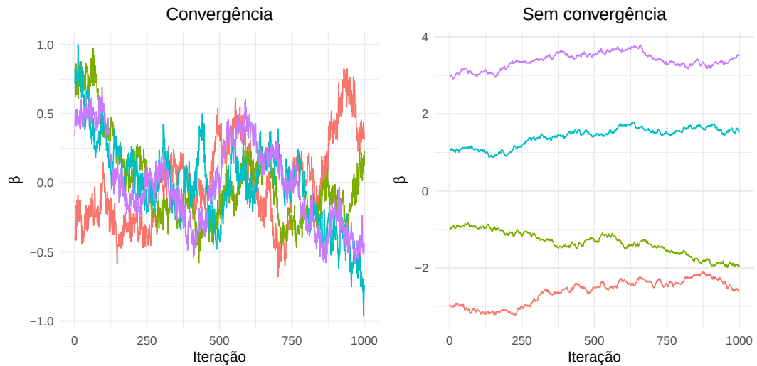
Figura 5: Exemplo ilustrativo de traceplots. À esquerda, cadeias convergidas apresentam boa mistura e exploram a mesma distribuição posteriori. À direita, cadeias não convergidas permanecem separadas, indicando problemas de convergência.
