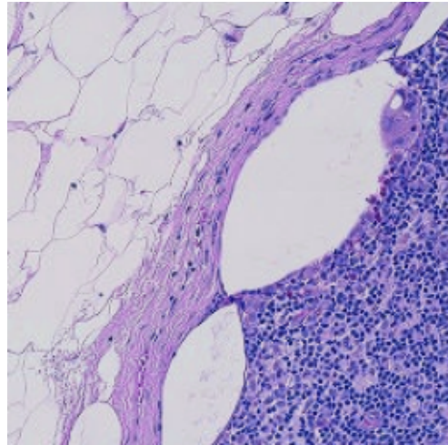
Jitter
