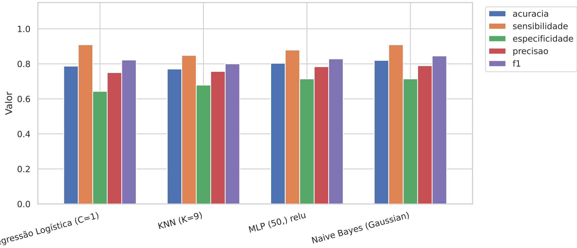
Comparação de Métricas — Regressão Logística vs KNN vs MLP vs Naive Bayes
