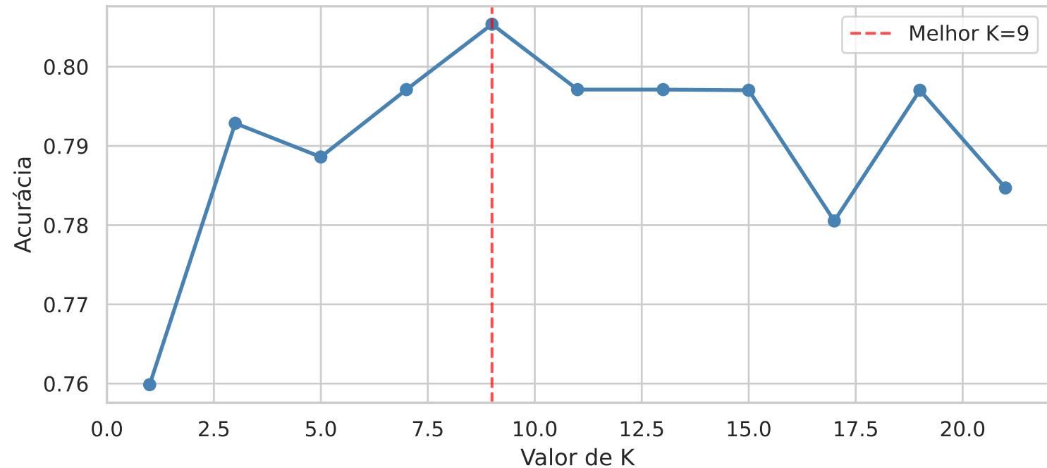
KNN — Acurácia por Número de Vizinhos
