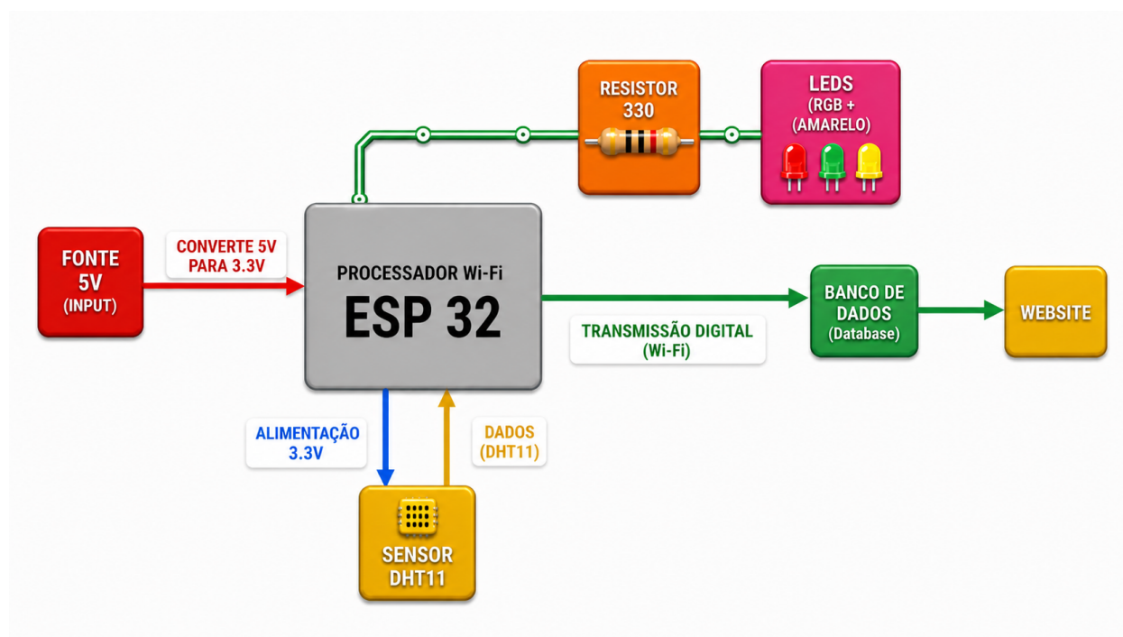
Figura 4: Diagrama de blocos do sistema de monitoramento ambiental com ESP32 e DHT11.
