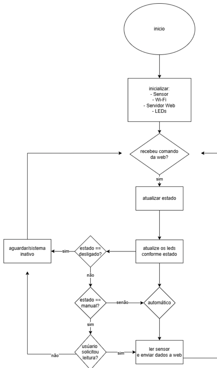
Figura 3: Fluxograma do software do leitor de temperatura
