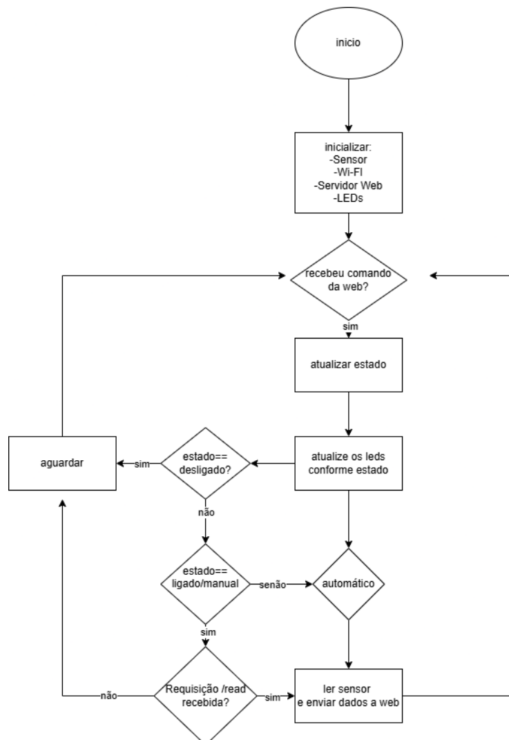
Figura 7: Fluxograma do software do leitor de temperatura
