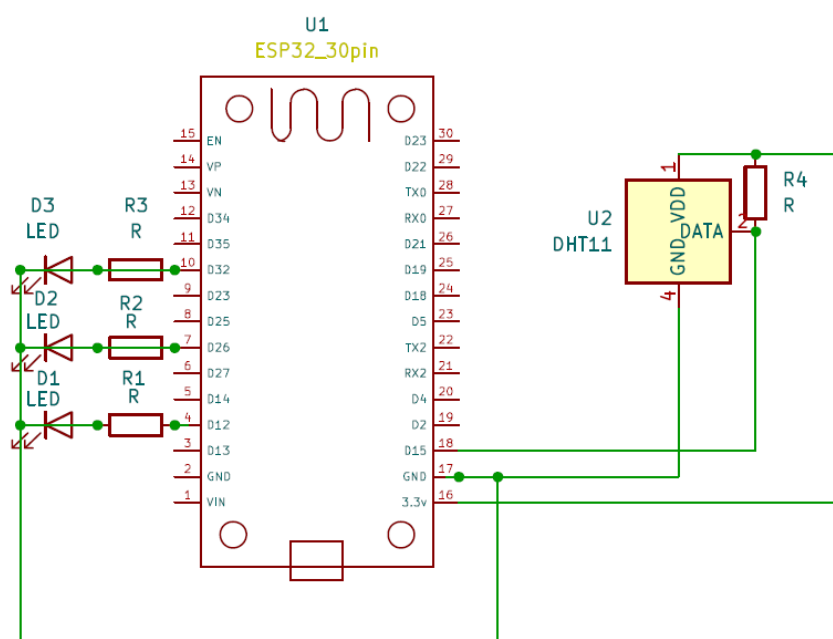
Figura 3: Esquemático com ESP32 e DHT11.
