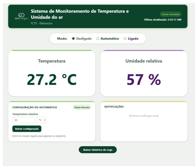
Figura 4: Protótipo de alta fidelidade da interface do usuário (versão Celsius)
