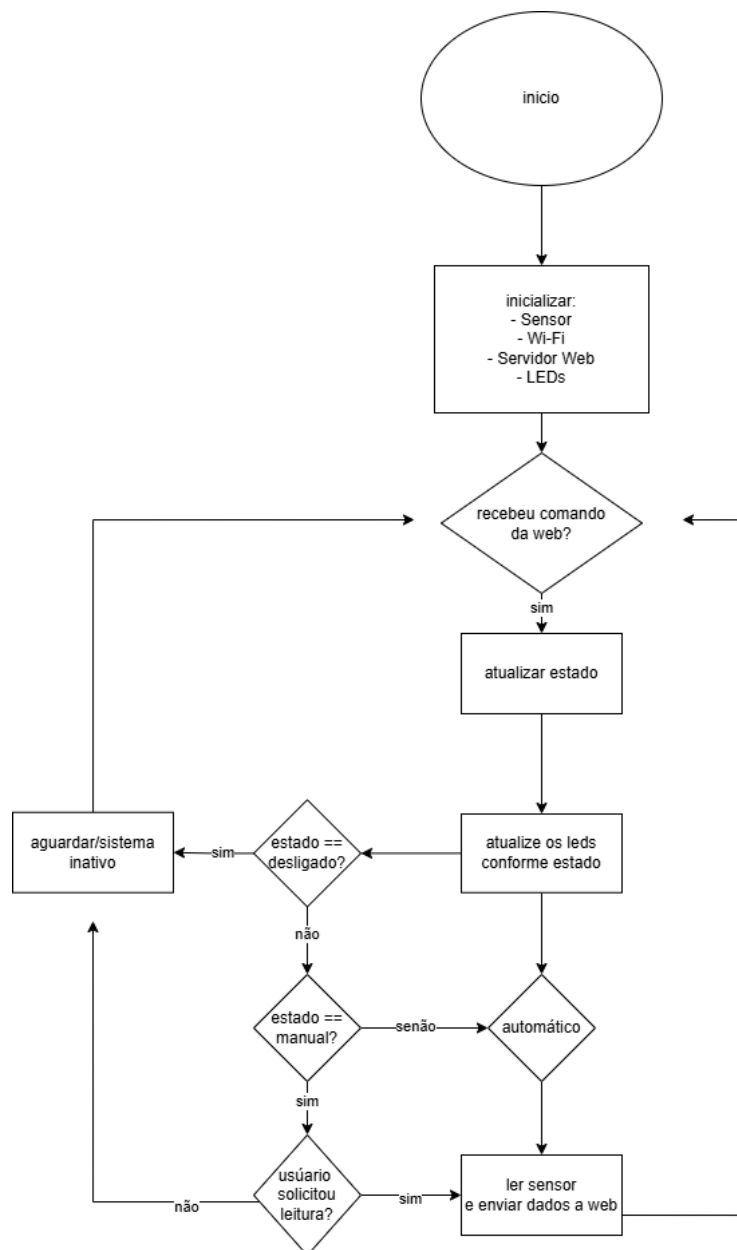
Figura 6: Fluxograma do software do leitor de temperatura
