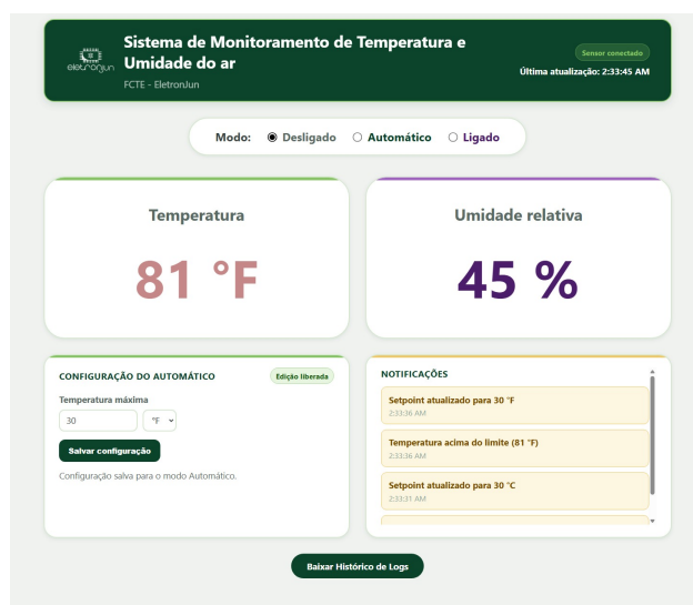
Figura 5: Protótipo de alta fidelidade da interface do usuário (versão Fahrenheit)
