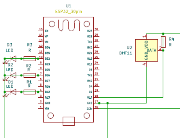
Figura 3: Esquemático com ESP32 e DHT11.
