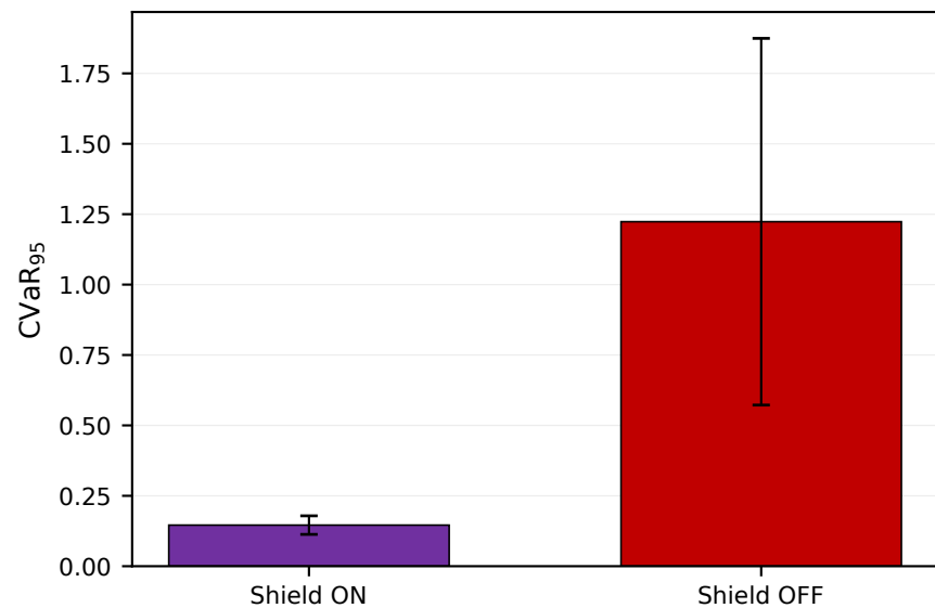
(d) CVaR 95
