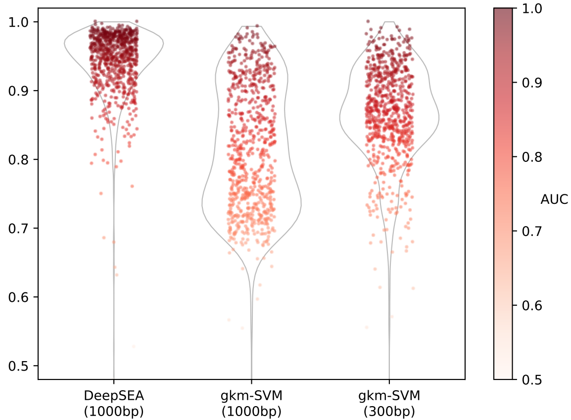
AUC
