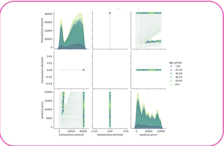
Pairplot
