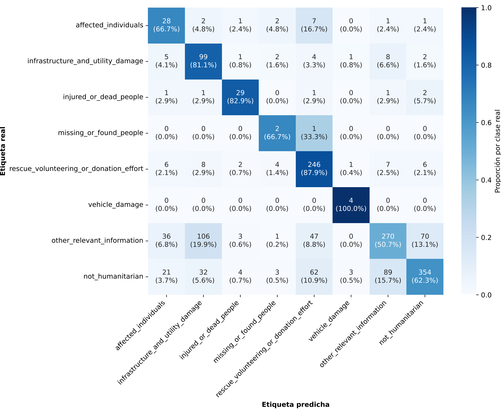
Matriz de confusión - BERTweet + Focal Loss
