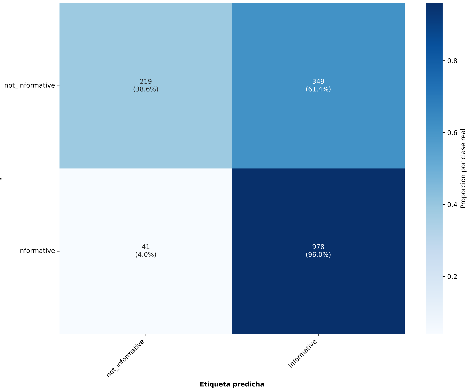
Matriz de confusión - Bi-LSTM
