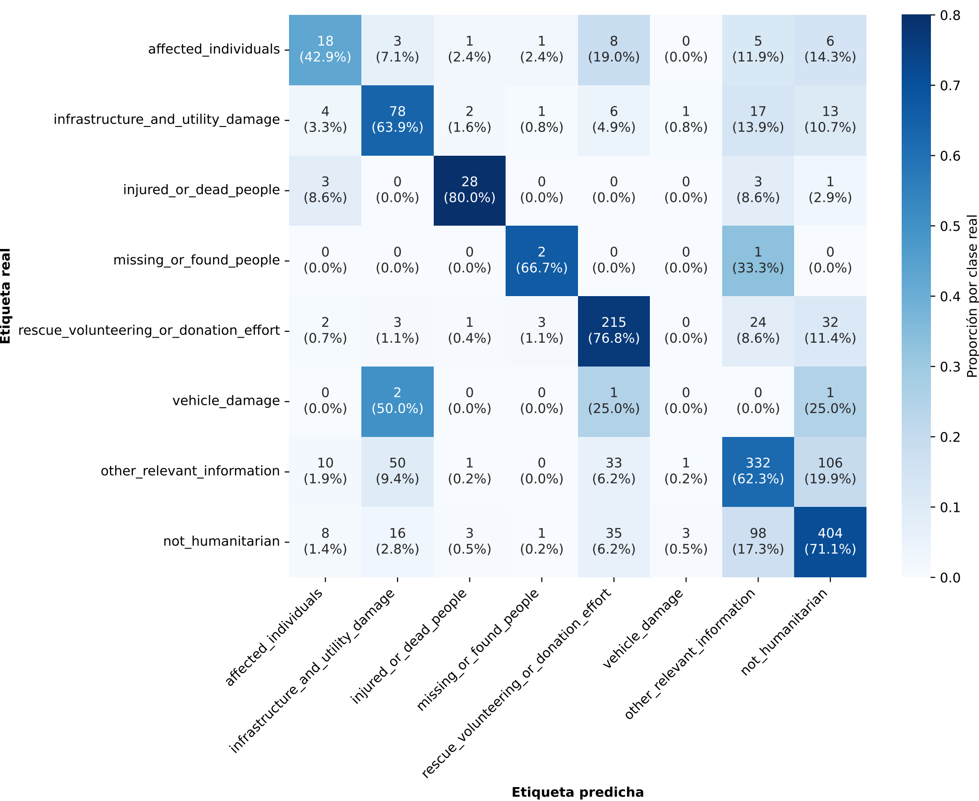
Matriz de confusión - Ensemble ponderado
