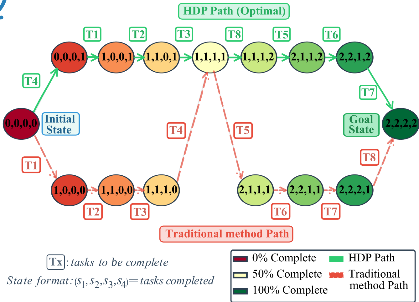
(D) DES Task Scheduling via DP
