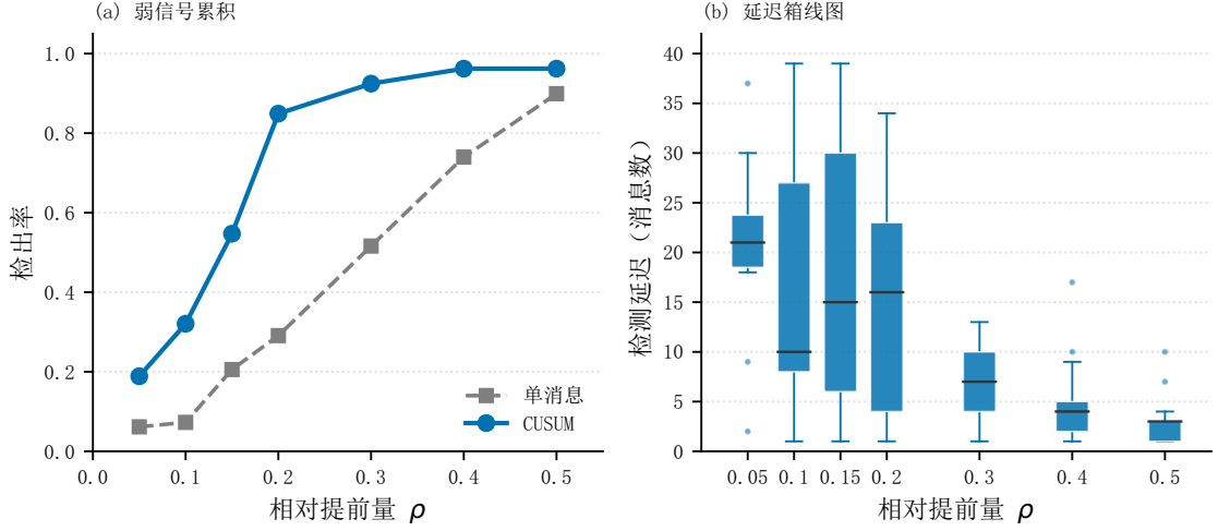
Fig. 12. CUSUM 相对单消息阈值的功效, 以及检测延迟箱线图。分层校准集上以参数化左尾 p 值驱动, 门限对应 ARL_0 = 500 , 延迟预算 40 条, 53 条测试子流。箱线只含预算内检出的注入; 未检出为删失, 见主表净检出率。
