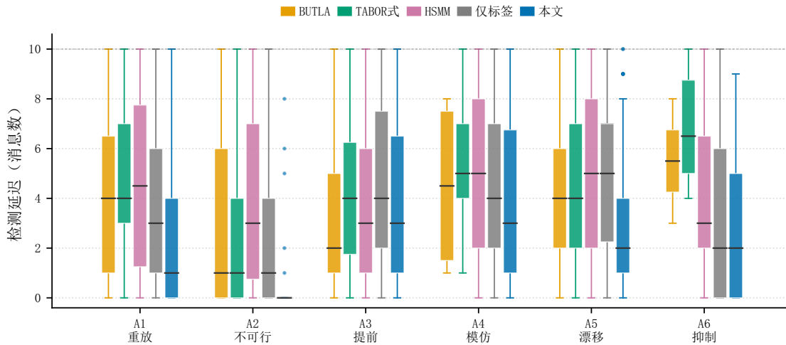
Fig. 8. \alpha = 0.01 、延迟预算 10 条下,各方法在六类攻击上的检测延迟(消息数)。箱线仅含预算内检出;未检出见净检出率。
