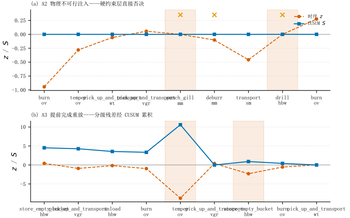
Fig. 3. A2 硬约束层否决与 A3 时序证据累积的逐条解析。阴影列为注入消息; 叉号表示硬约束层触发。
