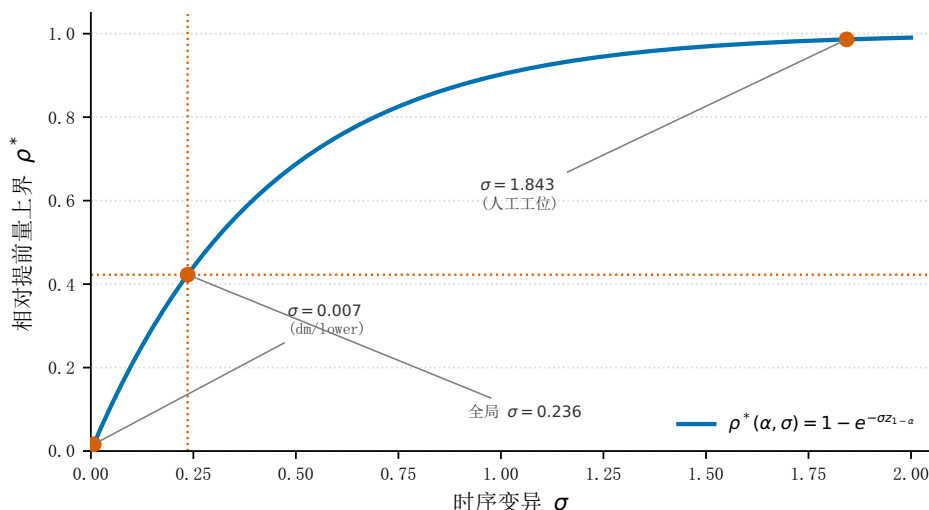
Fig. 5. \alpha = 0.01 单侧下 \rho^* 随 \sigma 的变化。标注点为低变异工序、全局加权 \sigma 与人工工位。
