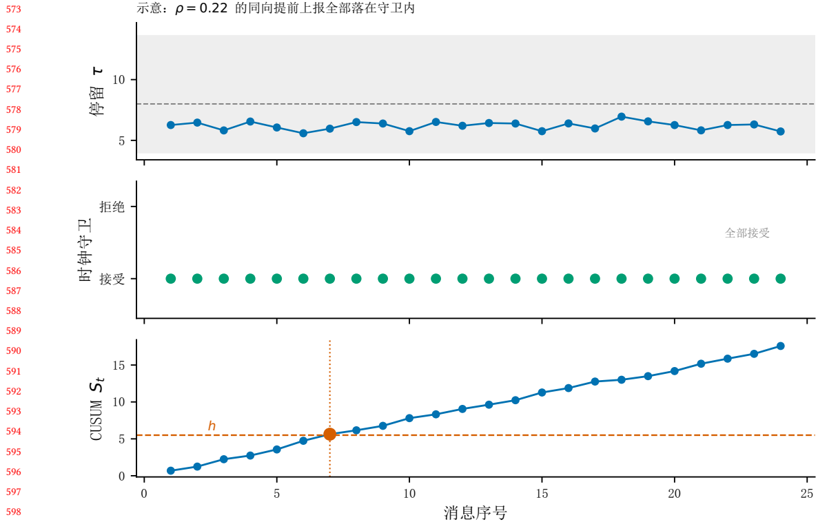
Fig. 4. 时钟守卫与分布型残差的差别(示意, 非评测轨迹)。灰色带为区间守卫; 同向提前上报全部被接受, CUSUM 仍累积越过 h 。
