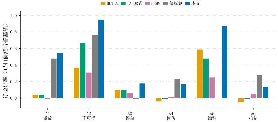
Fig. 7. \alpha = 0.01 、延迟预算 10 条、已扣除偶然告警基线的净检出率。仅标签为马尔可夫消融,而非独立的先行方法。
