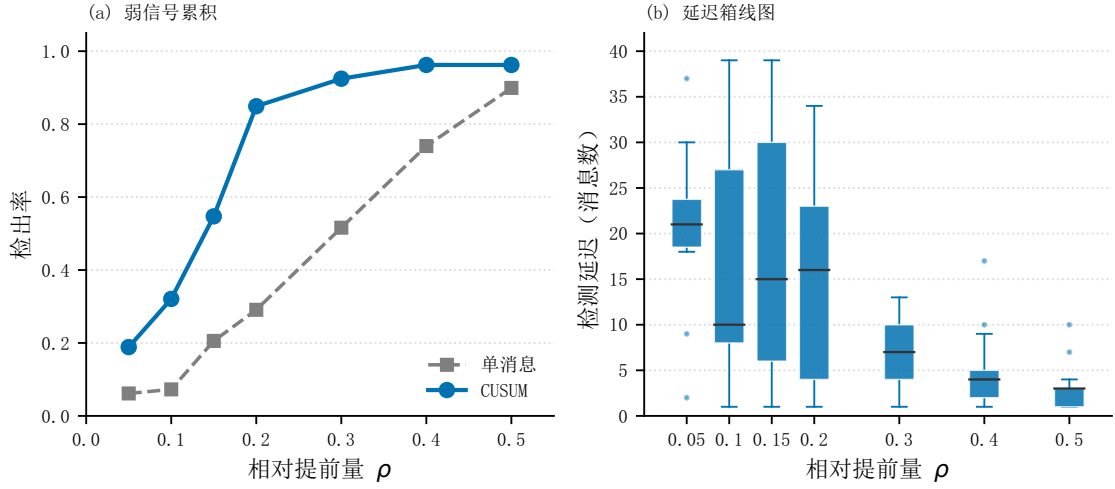
Fig. 12. CUSUM 相对单消息阈值的功效, 以及检测延迟箱线图。分层校准集上以参数化左尾 p 值驱动, 门限对应 ARL_0 = 500 , 延迟预算 40 条, 53 条测试子流。箱线只含预算内检出的注入; 未检出为删失, 见主表净检出率。
