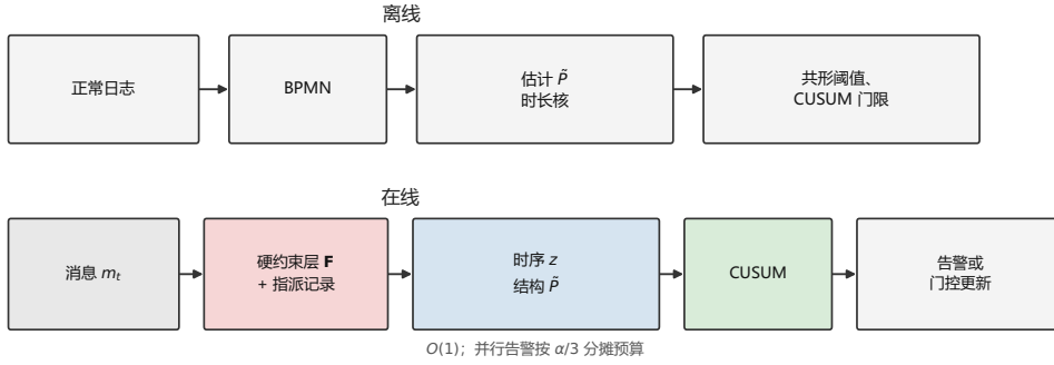
Fig. 2. 离线拟合与在线三路并行判决。硬约束层位于统计通道之前, 以免不可行样本污染校准。
