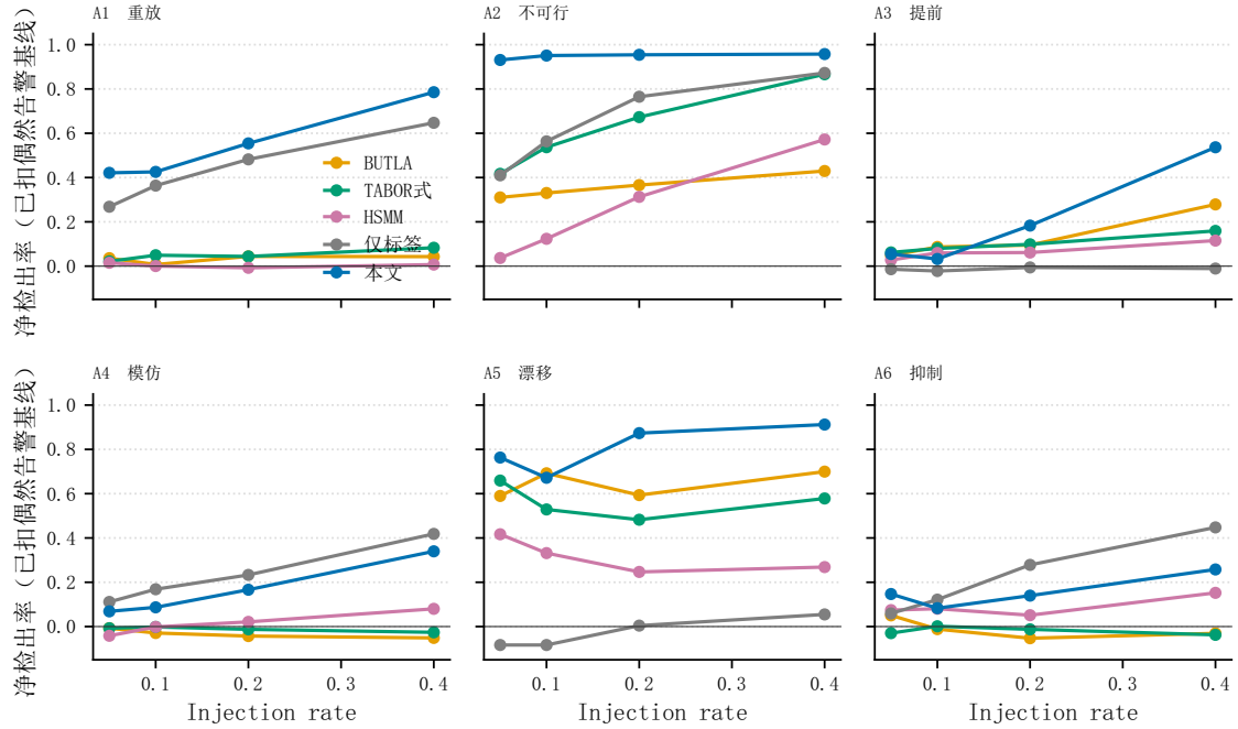
Fig. 9. 净检出率随注入率(5%~40%)的变化。按攻击族分设子图,可据此判断结论是否随攻击密度升高而失效。
