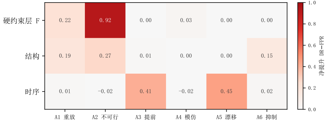
Fig. 6. 三路生产通道相对良性误报的净提升(DR-FPR)。A2 由硬约束层覆盖, A3/A5 仅时序通道有实质提升, A4 不存在专属通道。
