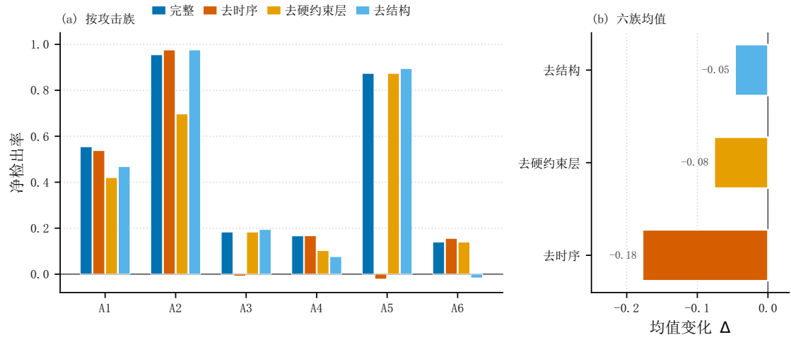
Fig. 10. 生产三路的消融( \alpha = 0.01 , 每路误报预算固定, 三个注入种子均值, 已扣除偶然告警基线)。去掉时序后 A3/A5 归零; 去掉硬约束层的降幅集中在 A2/A1, 去掉结构的降幅集中在 A6/A4。
