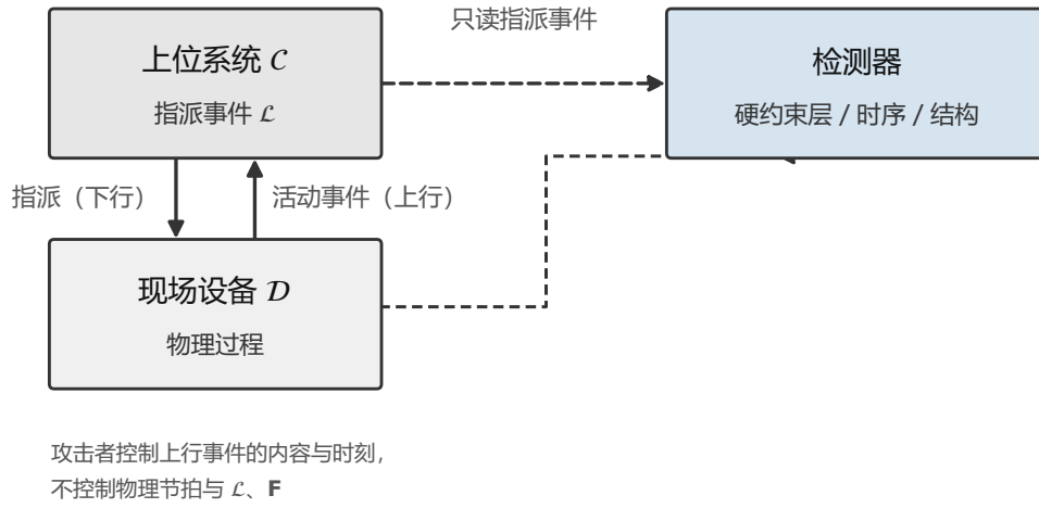
Fig. 1. 指派/事件回环。检测器只读取同一日志中的指派事件与参考模型可行性掩码,对上行事件逐条作在线判决。
