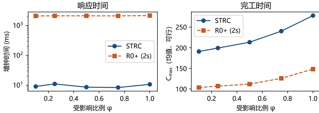
Fig. 9. 扰动规模扫描 (congested_8x4x4, 10 个随机种子): 有界修复与 R0+ 的算法耗时 (对数轴) 与完工时间随 \phi 变化。曲线取逐档均值, 离散度口径与表 12 同 (四分位距); 耗时一侧全扫描极差 2.2–23.8 ms, 始终在十毫秒量级, 这是本节结论所依据的唯一结果。
