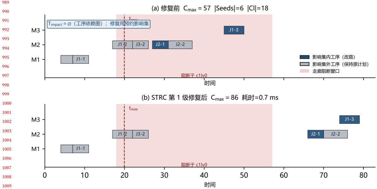
Fig. 6. 案例甘特图 (example_3x3x2, 随机种子 42)。 (a) 阻断前原排程，按是否属于 CI 着色； (b) 第 1 级修复后。工序依赖图上的影响域为空；蓝色工序对应影响集内运输被改路。本图仅示意局部改动的形态。
