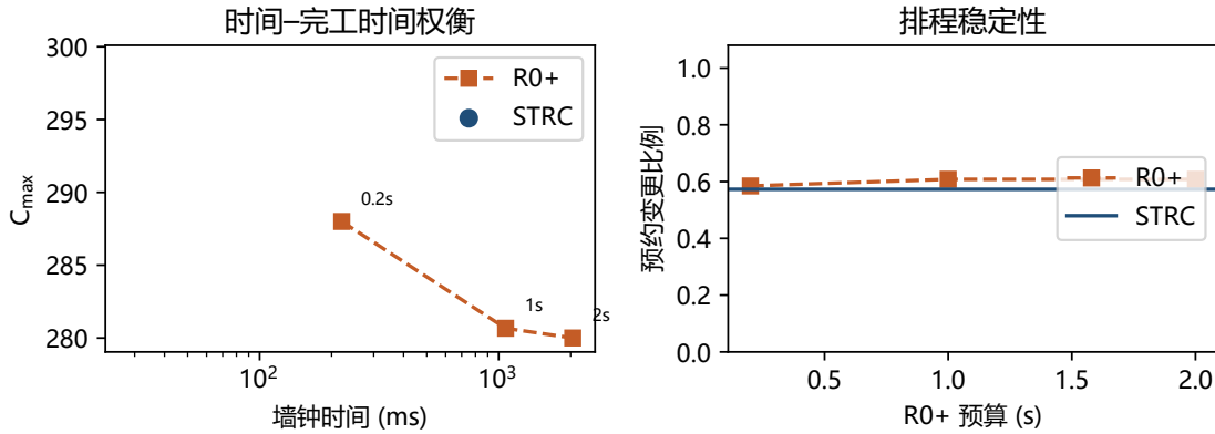
Fig. 7. E5: 不改写已结束占用的 R0+ 预算扫描与有界修复结果 (congested_8x4x4, 3 个随机种子均值)。左: 算法耗时- C_{\max} , 两条曲线不相交; 右: 占用改动比例, 两法均约为 0.6。
