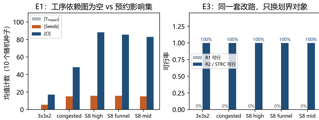
Fig. 5. E1/E3 扩样可视化 (5 算例 \times 10 个随机种子均值)。左: 工序依赖图上的影响域为空, 而起点占用与预约影响集非空; 柱高为每算例 10 格的均值, 离散度按四分位距见表 4 ( |C| 的 IQR 逐算例在 2–8 之间, 影响域一组恒为零故无离散度)。右: 同一套改路、只换划界对象时 R1 可行率为 0、R2 为 100%; 该幅为逐格计数 (各 50 格), 故不给出离散度。
