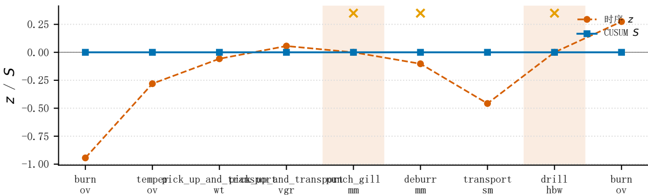
(b) A3 抢跑重放——分级残差经 CUSUM 累积
