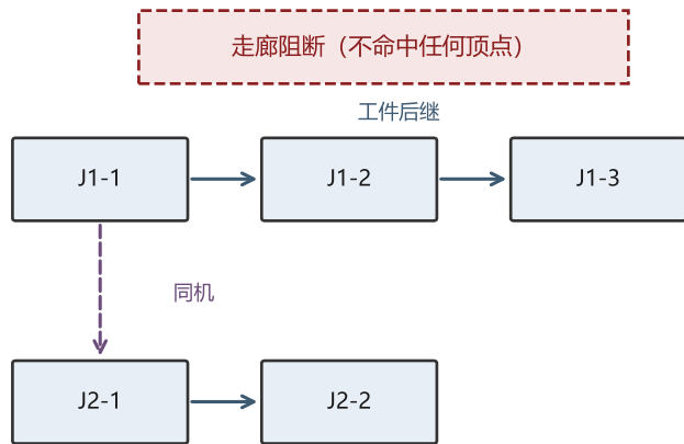
(a) 任务依赖图 G_T (顶点 = 工序)
