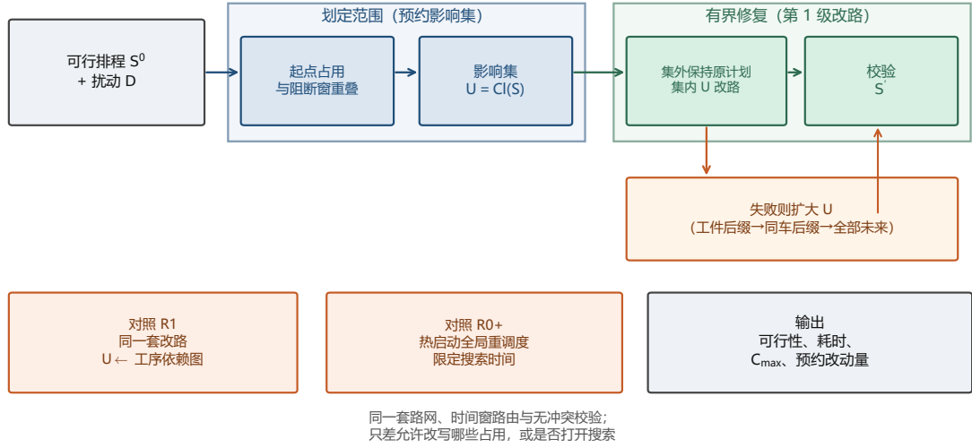
Fig. 4. 按预约影响集划界的有界恢复。上排: 由起点占用得到影响集并改路; 中排: 失败后扩大允许改写的范围; 下排: 按工序依赖图划界的对照与热启动全局重调度对照, 以及输出指标。本图只画方法层的三条路径; 毫秒档内另有三条对照 (第 6.9 节)。
