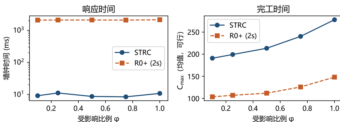
Fig. 9. 扰动规模扫描 (congested_8x4x4, 10 个随机种子): 有界修复与 R0+ 的算法耗时 (对数轴) 与完工时间随 \varphi 变化。曲线取逐档均值, 离散度口径与表 12 同 (四分位距); 耗时一侧全扫描极差 2.2–23.8 ms, 始终在十毫秒量级, 这是本节唯一据以立论的读数。
