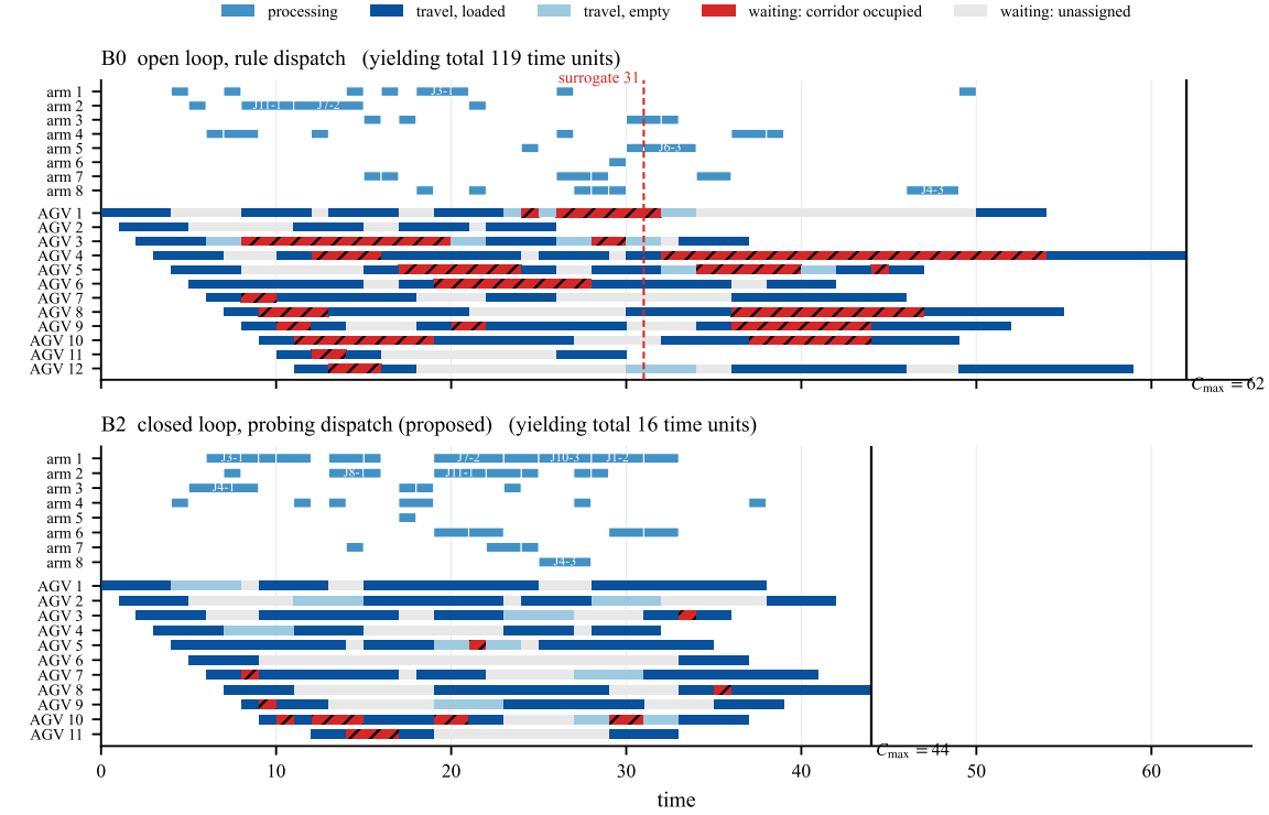
Fig. 8. 同一漏斗算例上 B0(上) 与 B2(下) 的解。机械臂与车辆共用时间轴; 车辆行区分空载段、满载段, 以及两类等待——按成因分开着色是本图唯一要紧的设计: 同一运输任务两段之间的空隙是车被前方占用的走廊拦在停靠位上, 即让行, 也就是本文所处理的那种延误; 不同任务之间的空隙则是车无活可干, 属于车队规模的症状。两者若同色, 读者就会把其中一种归因成另一种。图内文字为英文以便与代码输出一致。
