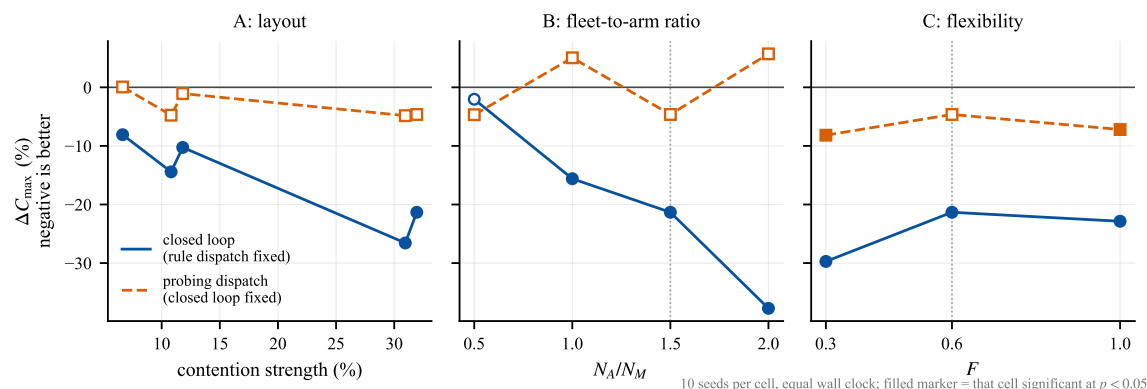
Fig. 4. 两个主效应在三个因子族上的分布。左: 布局族, 横轴为争用强度; 中: 车臂比族, 横轴为 N_A/N_M ; 右: 柔性族。B 与 C 两族含共用基点 (空心竖线所在的 1.5 与 0.6), 它同时列于 A 族的 A funnel。实心标记为该格自身显著 ( p < 0.05 ), 空心为不显著。闭环增益几乎处处显著且大体随争用上升; 试探增益只在柔性族两端显著, 在车臂比族的四个水平上符号交替、无一显著——因此本图要读的是两条曲线可信度的差别, 而不是试探那条曲线的形状。
