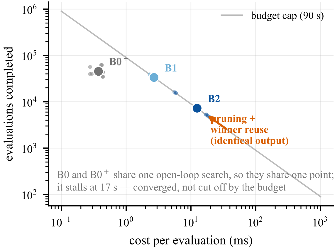
Fig. 6. 固定挂钟预算把“单次评价成本”与“完成的评价次数”锁成一条双曲线，灰线是各档共享的 90 秒预算上限。这就是本文反复引用的兑换率：一个机制必须在每次评价里买到的，多于它在评价次数上让出的。两个闭环配置贴在线上——它们每一次都把预算跑满；开环配置明显落在线下方，因为它在四百余代后不再改进而自行停止，约 17 秒即收敛，并非被预算掐断（第 5.1.2 小节）。B0 与 B0 + 共用同一次开环搜索，故共用一个点，差别只在执行方式。淡色小点是三个算例的逐个读数，实心大点取其几何平均——在对数轴上只有几何平均能保持“成本 × 次数 = 该档挂钟”这一关系。橙色箭头是降本消融的两档——它是唯一一种不改变输出就能沿该线移动的干预（命题 3），因此这一段位移是纯粹的算力节省。
