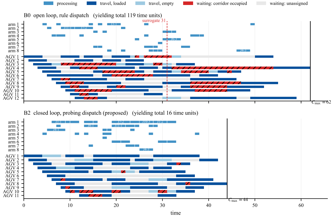
Fig. 8. 同一漏斗算例上 B0(上) 与 B2(下) 的解。机械臂与车辆共用时间轴; 车辆区分空载段、满载段, 以及两类等待——按成因分开着色是本图唯一要紧的设计: 同一运输任务两段之间的空隙是车被前方占用的走廊拦在停靠位上, 即让行, 也就是本文所处理的那种延误; 不同任务之间的空隙则是车无活可干, 属于车队规模的症状。两者若同色, 读者就会把其中一种归因成另一种。图内文字为英文以便与代码输出一致。
