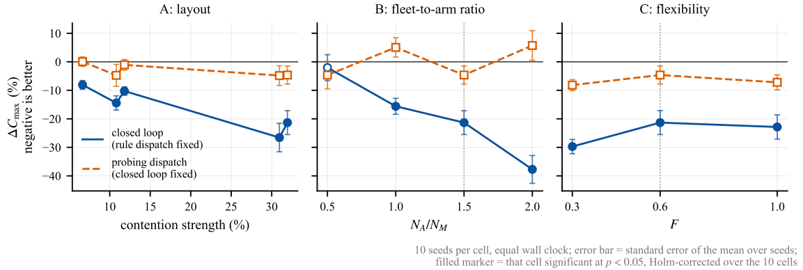
Fig. 4. 两个主效应在三个因子族上的分布。左: 布局族, 横轴为争用强度; 中: 车臂比族, 横轴为 N_A/N_M ; 右: 柔性族。B 与 C 两族含共用基点 (空心竖线所在的 1.5 与 0.6), 它同时列于 A 族的 A funnel。实心标记为该格在 Holm 校正后仍显著 ( p < 0.05 , 族为一个效应的 10 个格), 空心为不显著。误差棒为该格 10 个种子上逐对相对增益的均值标准误。闭环增益 9 格显著且大体随争用上升; 试探增益校正后无一格显著, 其误差棒逐格跨零, 在车臂比族的四个水平上符号还交替——因此本图要读的是两条曲线可信度的差别, 而不是试探那条曲线的形状。
