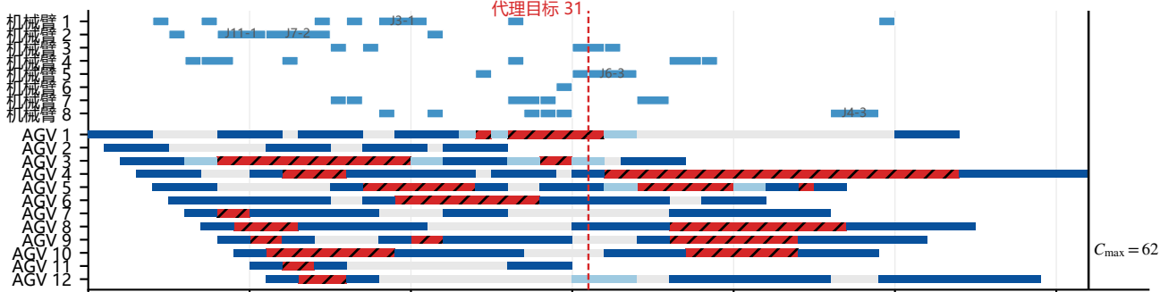
B0 开环, 规则派车 (让行合计 119 时间单位)
