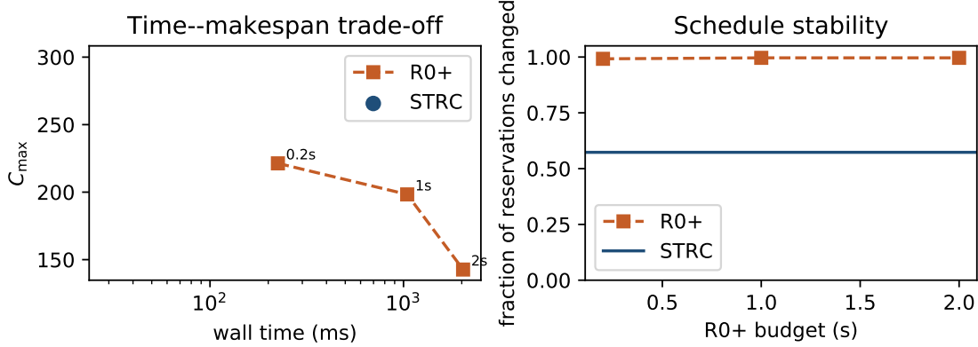
Fig. 6. E5: R0+ 预算扫描与 STRC 定点 (congested_8x4x4, 3 种子均值)。左: 耗时- C_{\max} , 两条曲线不相交; 右: 预约改动比例。
