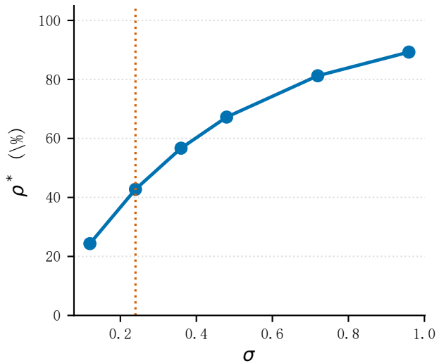
(b) 上界 \rho^*(\sigma)
