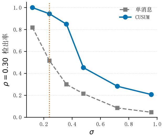
(a) 可检测性随 \sigma
