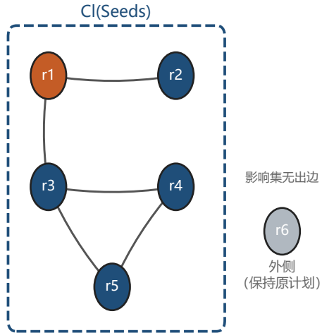
(b) 依赖边与预约影响集
